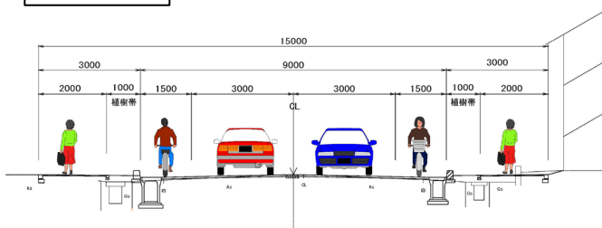
標準断面図
