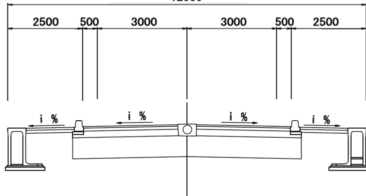
標準断面図
