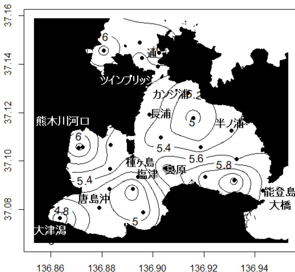
図 1. 海底付近の溶存酸素分布(mg/L) 【2026/7/29 観測】※●は観測点
