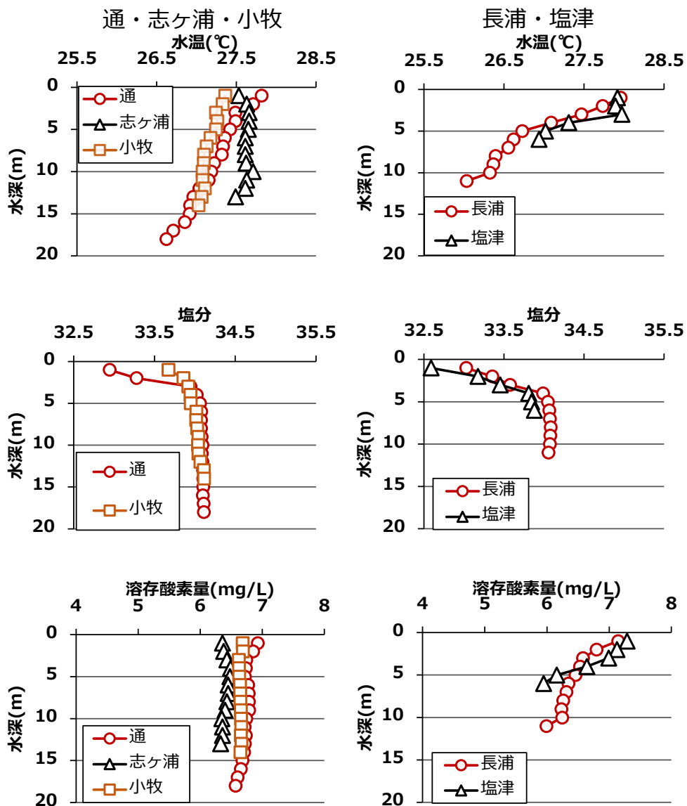
図2. 主な観測点の水温・塩分・溶存酸素の鉛直分布 【2026/7/29 観測】
