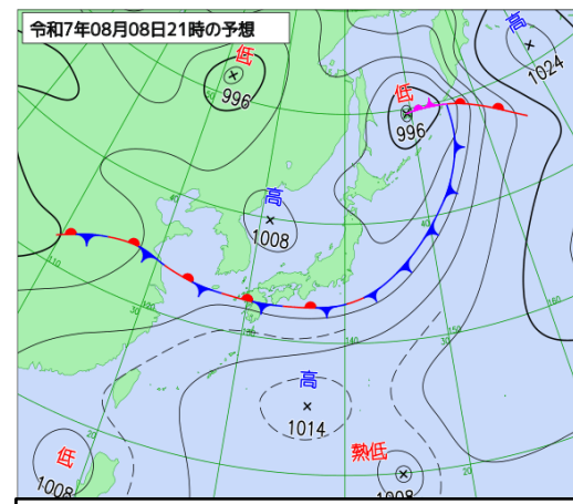
8日 21時 予想天気図
