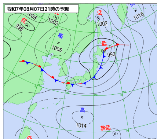
7日 21時 予想天気図
