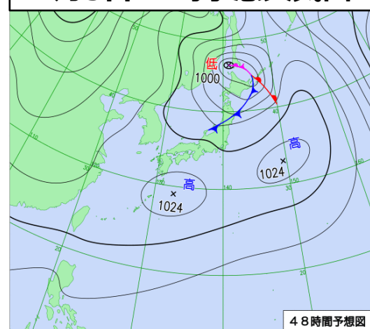
1月5日21時予想天気図
