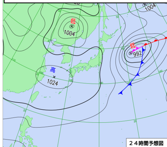
1月4日21時予想天気図
