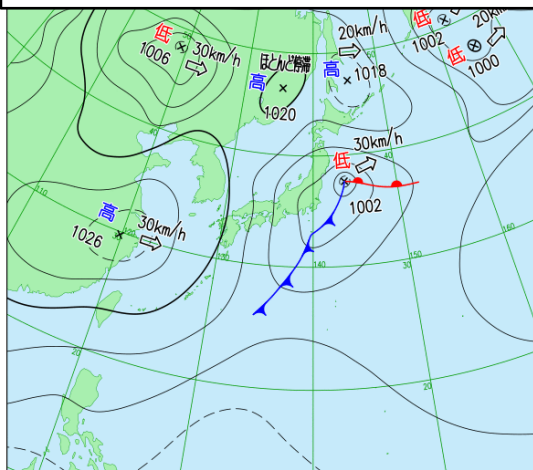
1月4日3時実況天気図
