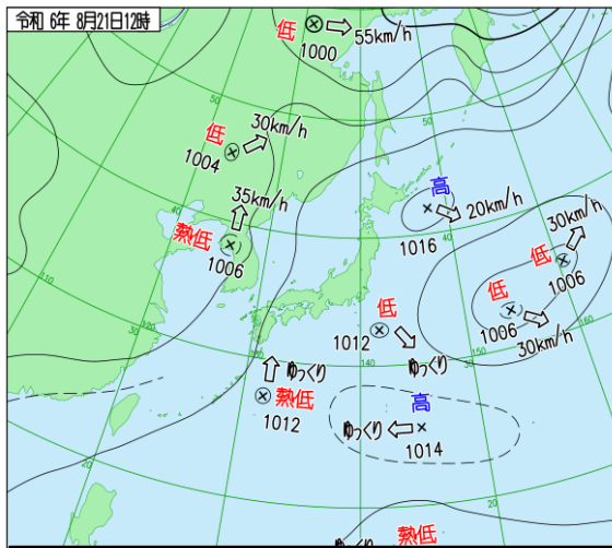
8月21日 12時 実況天気図
