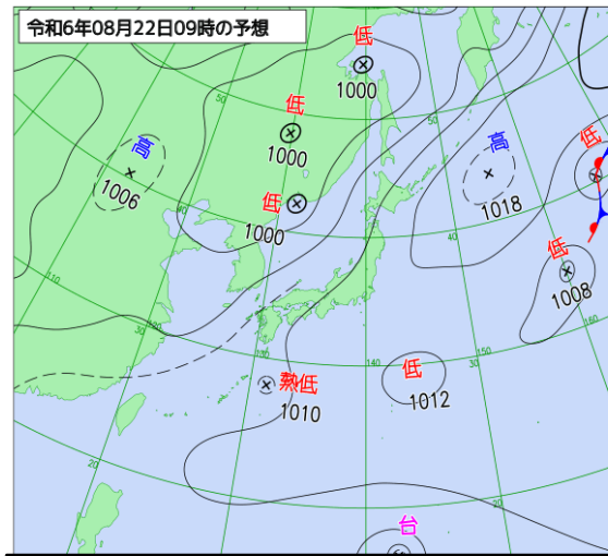
8月22日 9時 予想天気図
