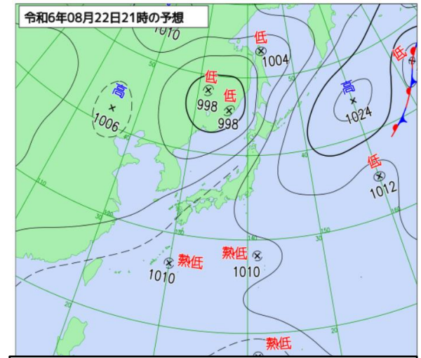
8月22日 21時 予想天気図
