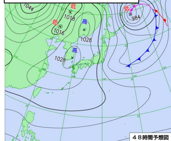
13日21時予想天気図
