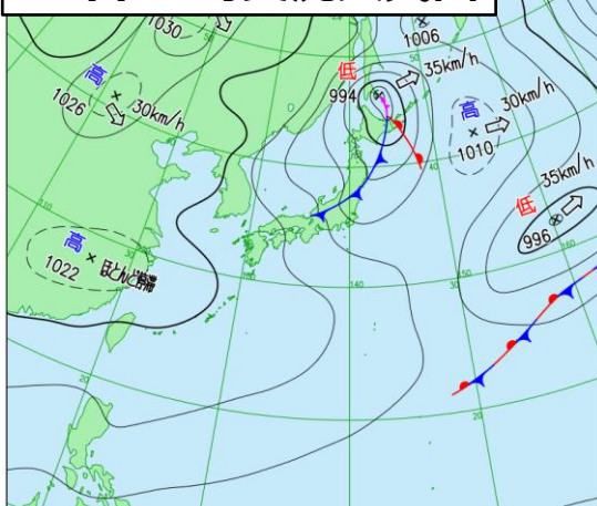
12日12時実況天気図
