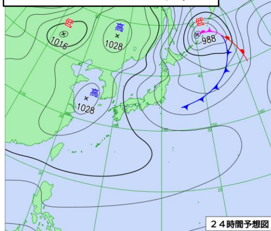
13日9時予想天気図
