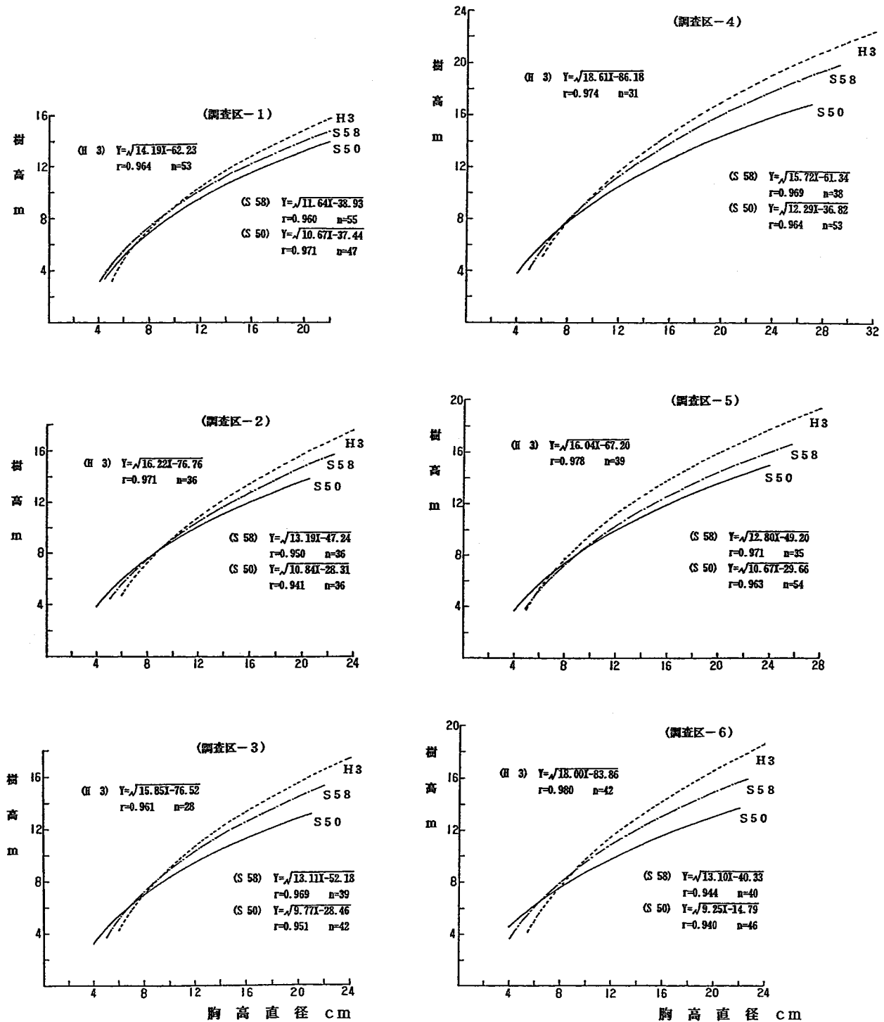
図-13 樹高曲線
