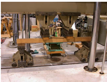
実大材曲げ強度試験
