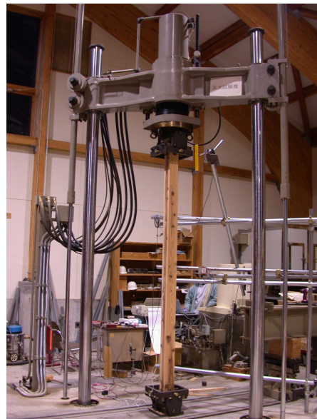
縦圧縮強度試験
