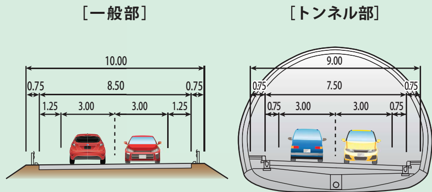
標準断面図 単位:m
