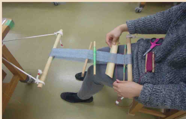
上下に分けた経糸の間に緯糸を通します。
