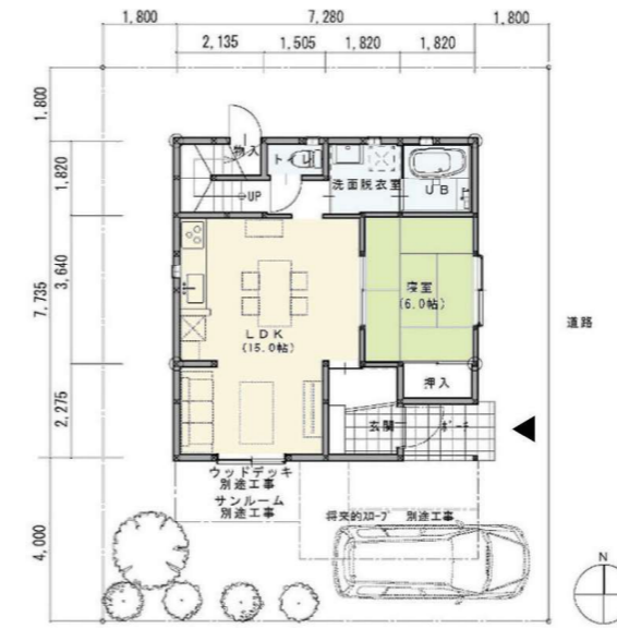
1階平面図
