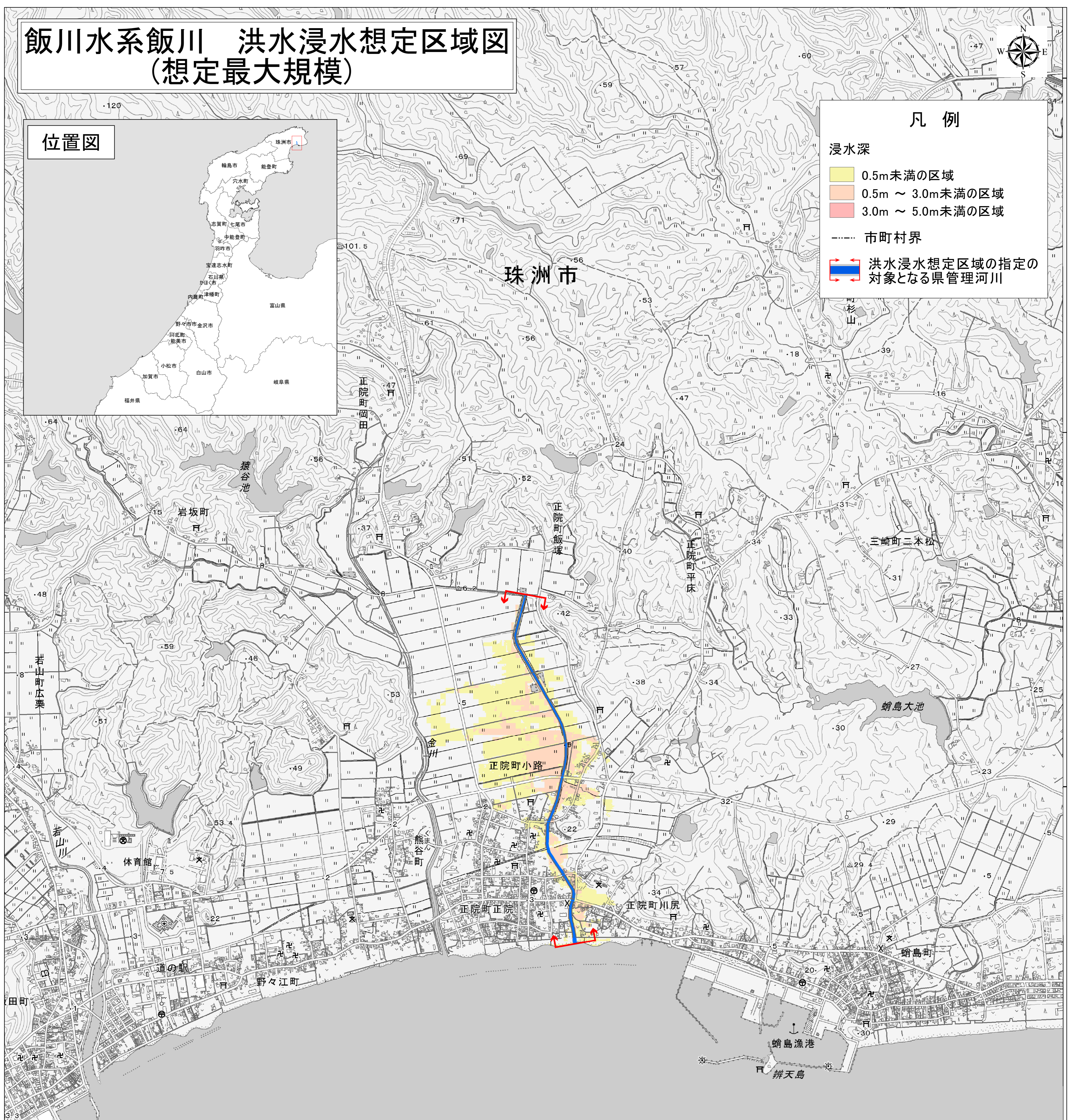
飯川水系飯川洪水浸水想定区域図 (想定最大規模)
