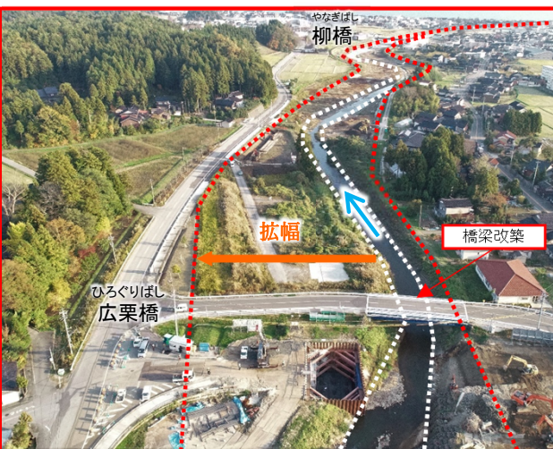
若山川における河川改修の実施（石川県）
