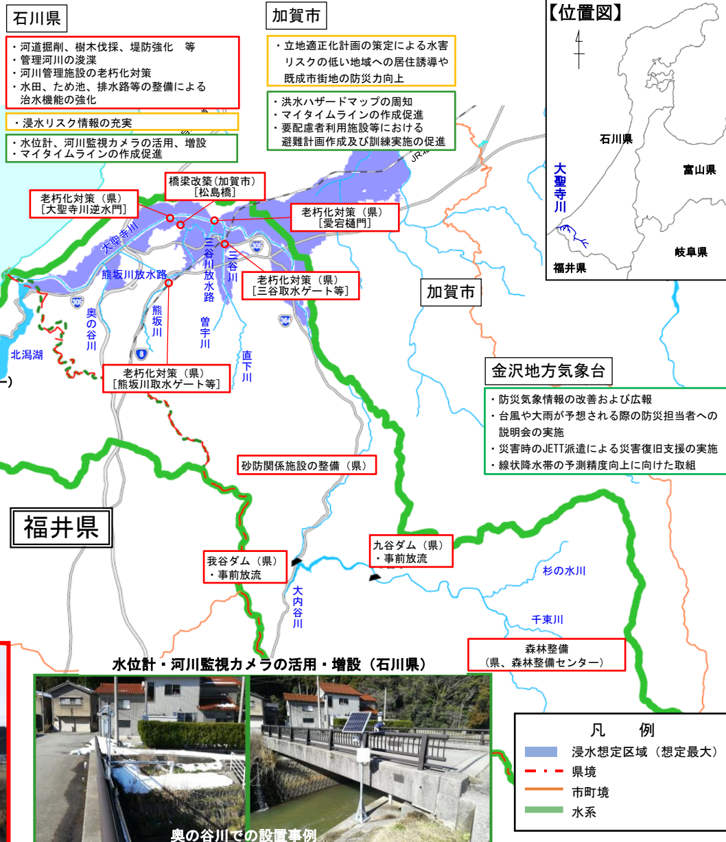
砂防関係施設の整備（石川県）
