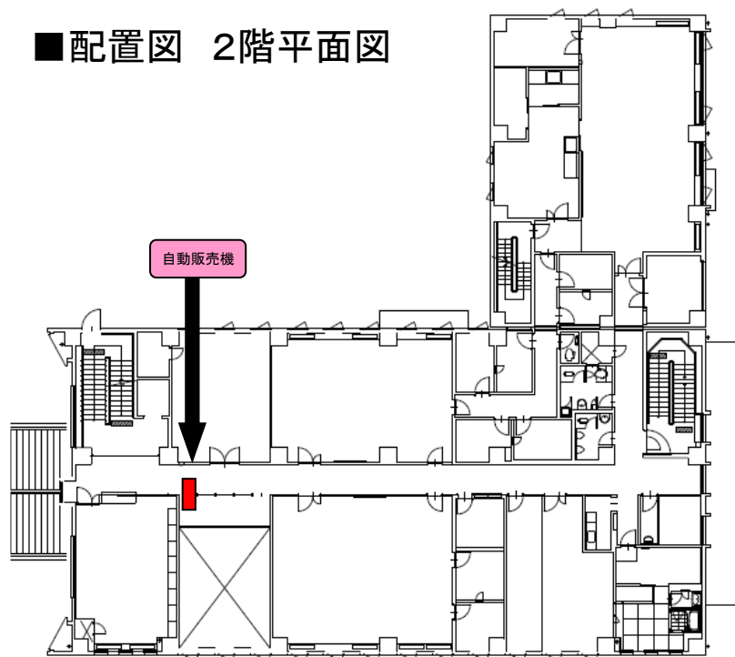
小松警察署 2階平面図
