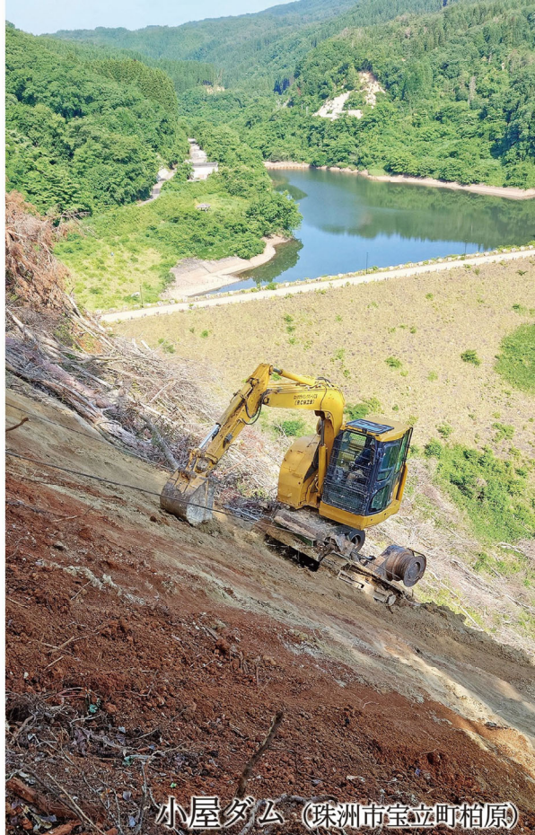
房田地すべり対策（輪島市房田町）
