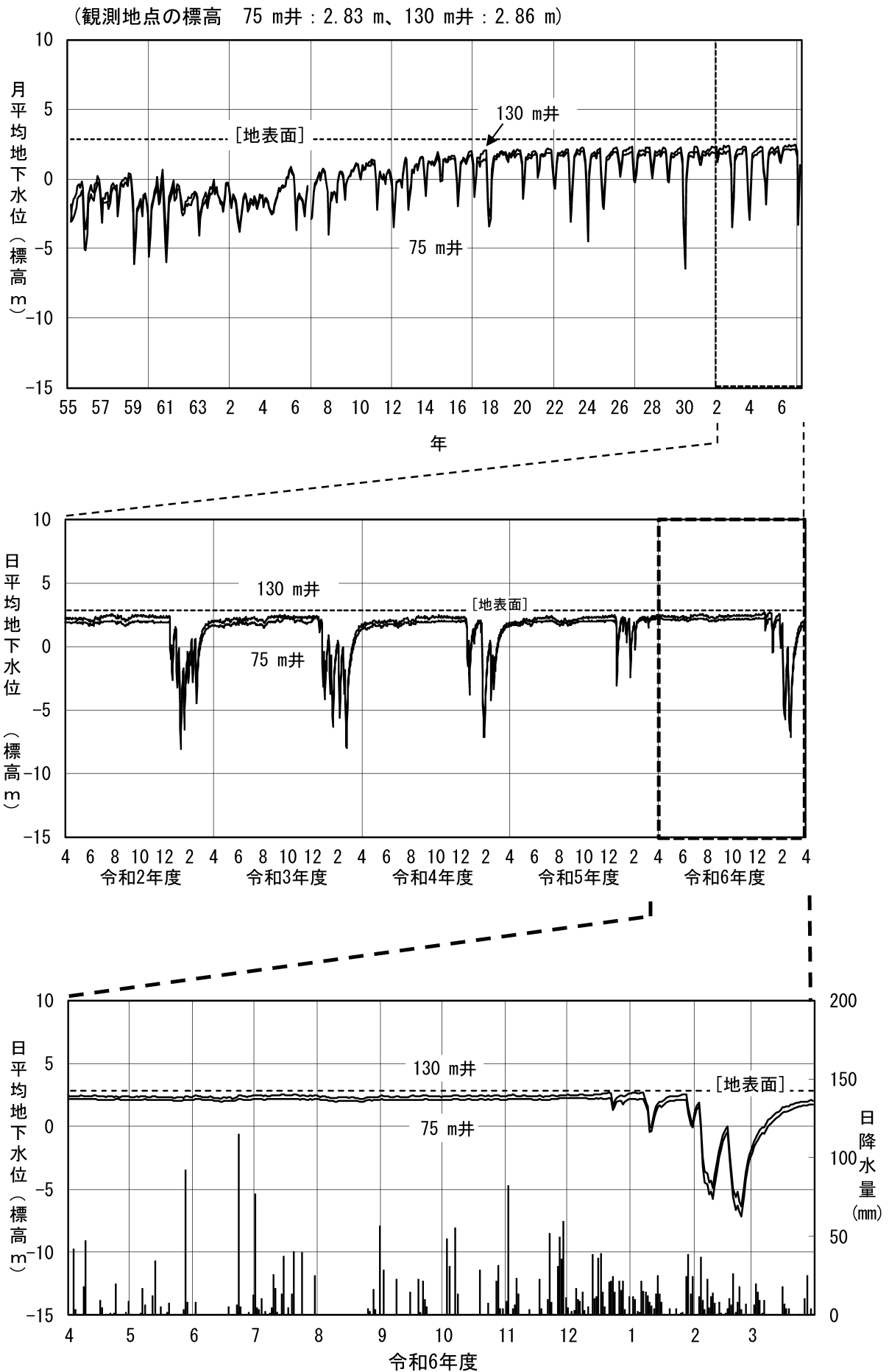
図 2-5 (3) 地下水水位変動図 (②金沢市須崎町)
