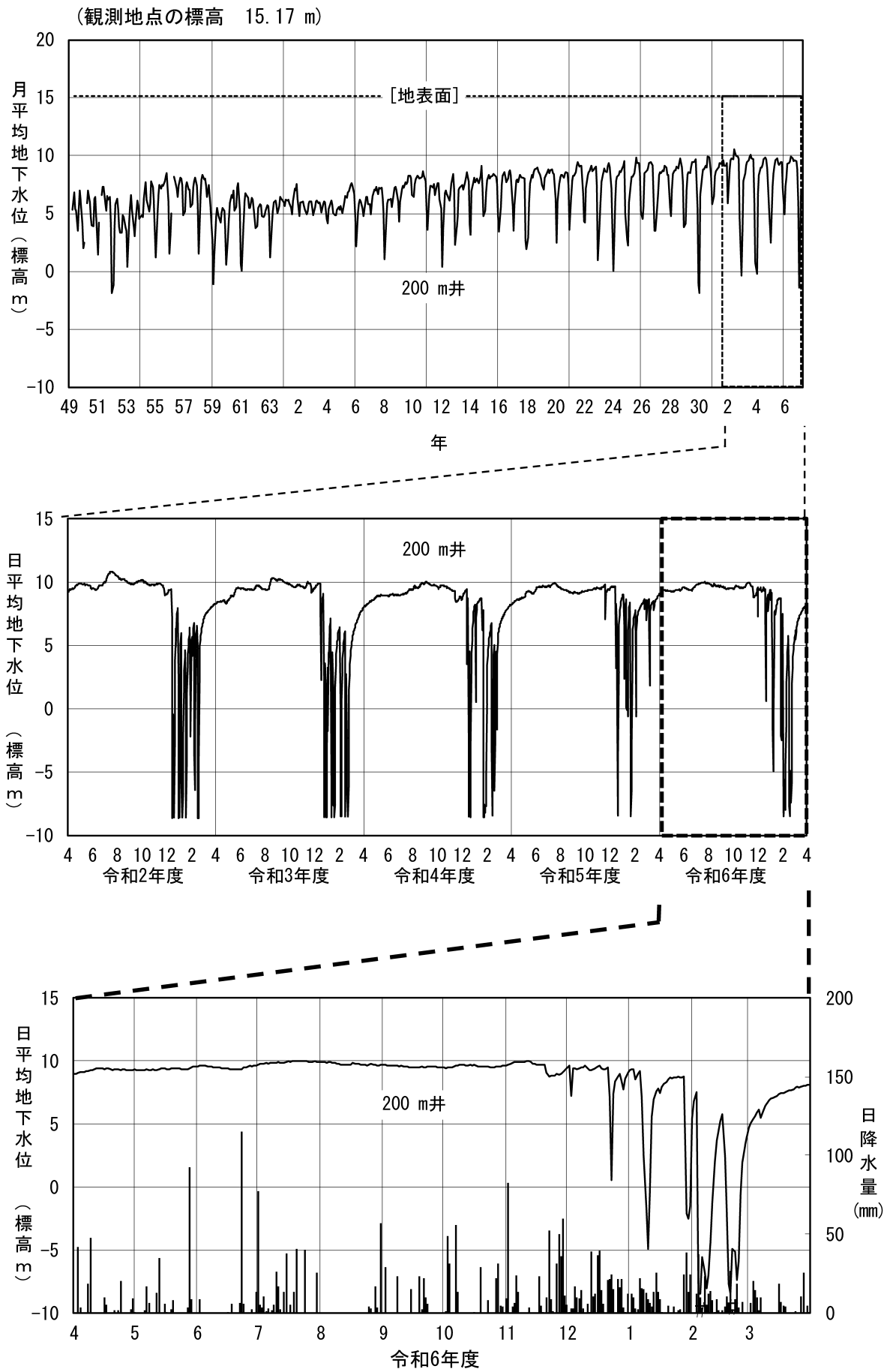
図 2-6(4) 地下水位変動図 (⑨金沢市長町)
