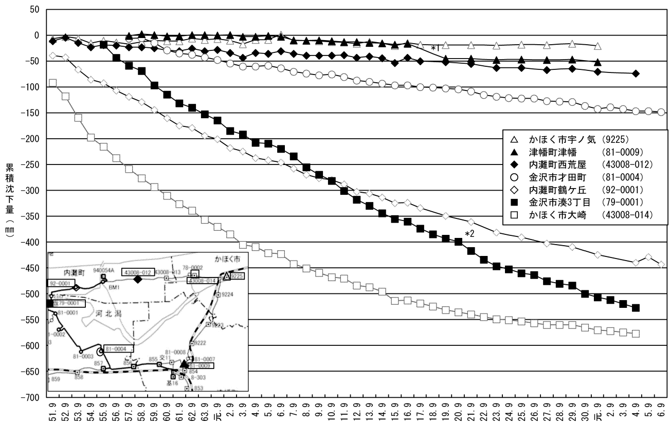
図 2-3(1) 主な水準点の累積地盤沈下量 (津幡町～金沢市)
