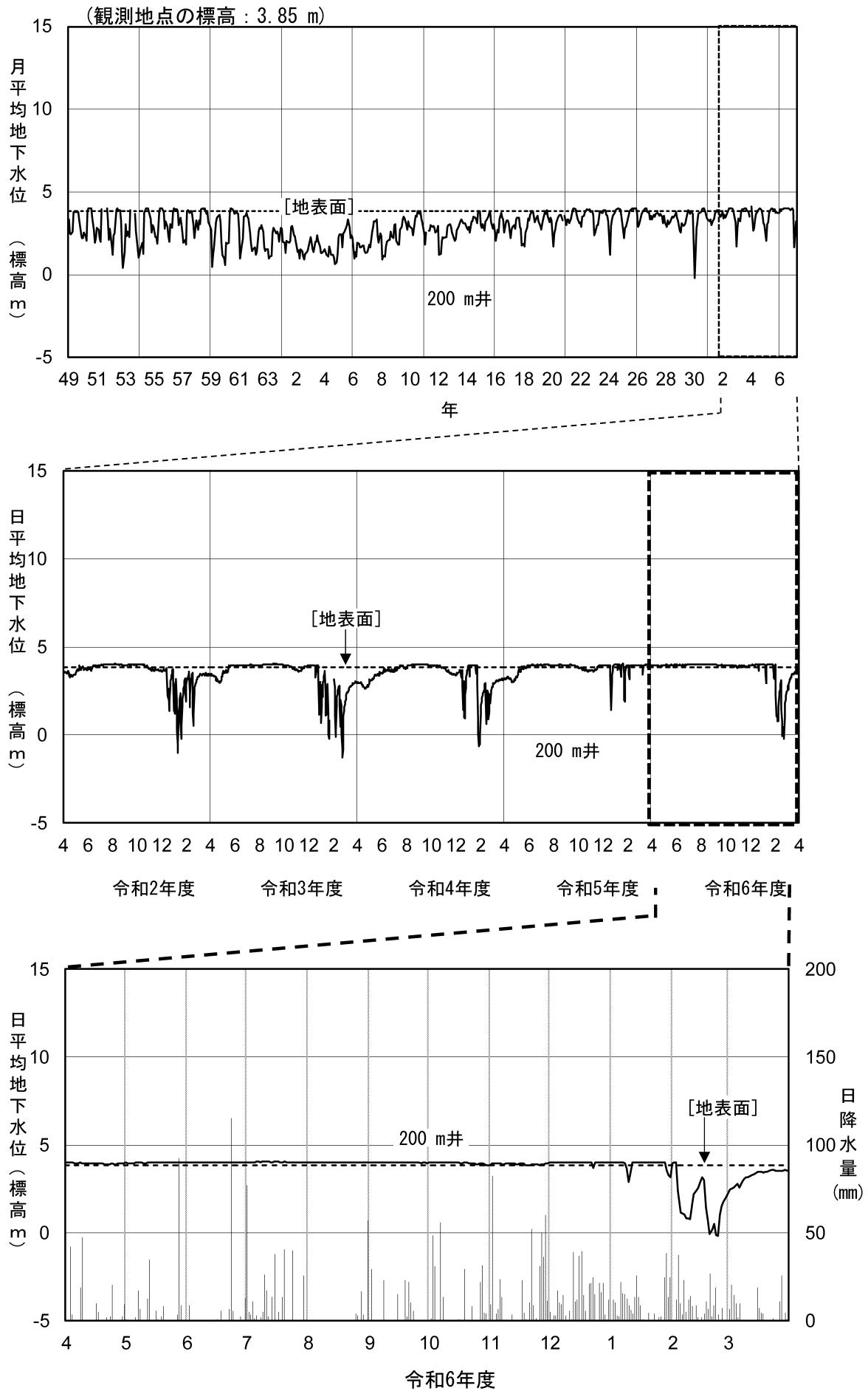
図 2-6(11) 地下水位変動図 (⑩金沢市福増町)
