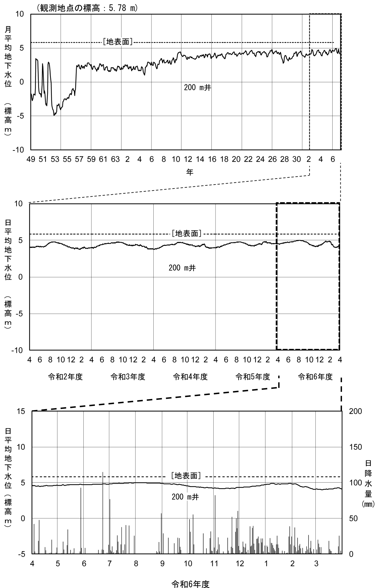
図 2-6(15) 地下水位変動図 (㊸白山市井関)
