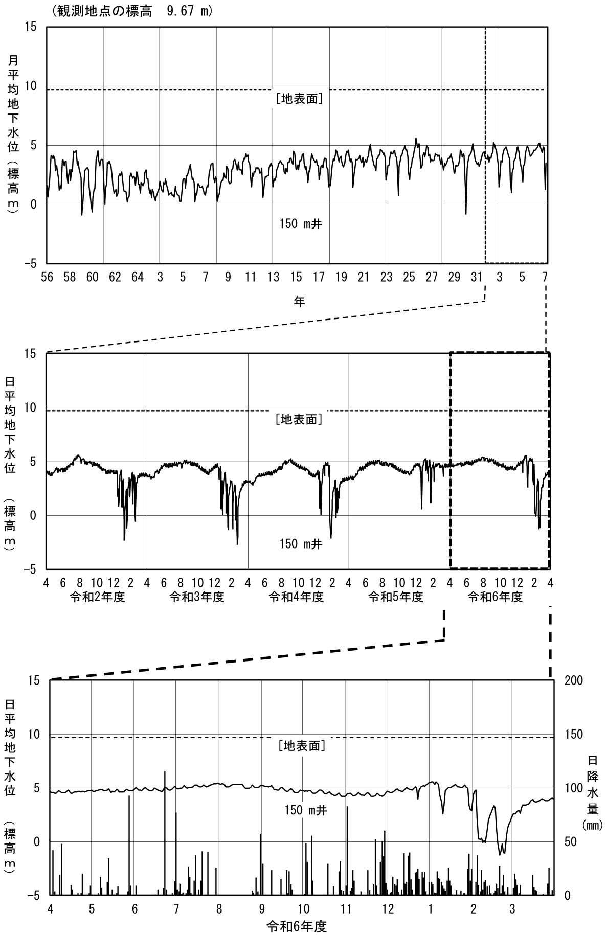
図 2-6 (5) 地下水位変動図 (⑩金沢市新保本町)
