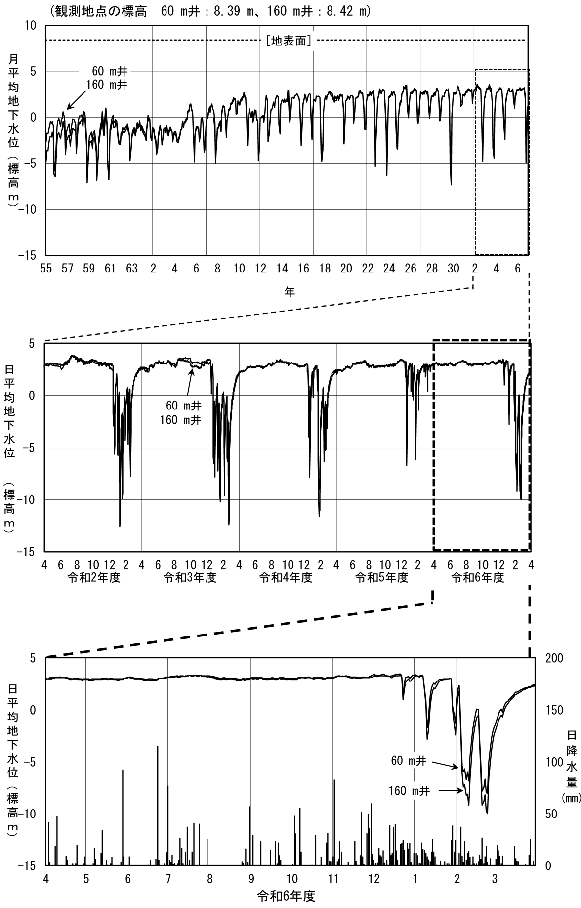
図 2-5 (5) 地下水位変動図 (③金沢市浅野本町)
