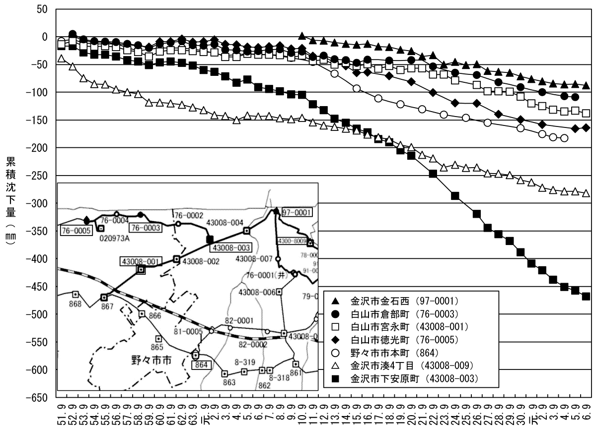
図 2-3(3) 主な水準点の累積地盤沈下量 (金沢市～白山市)
