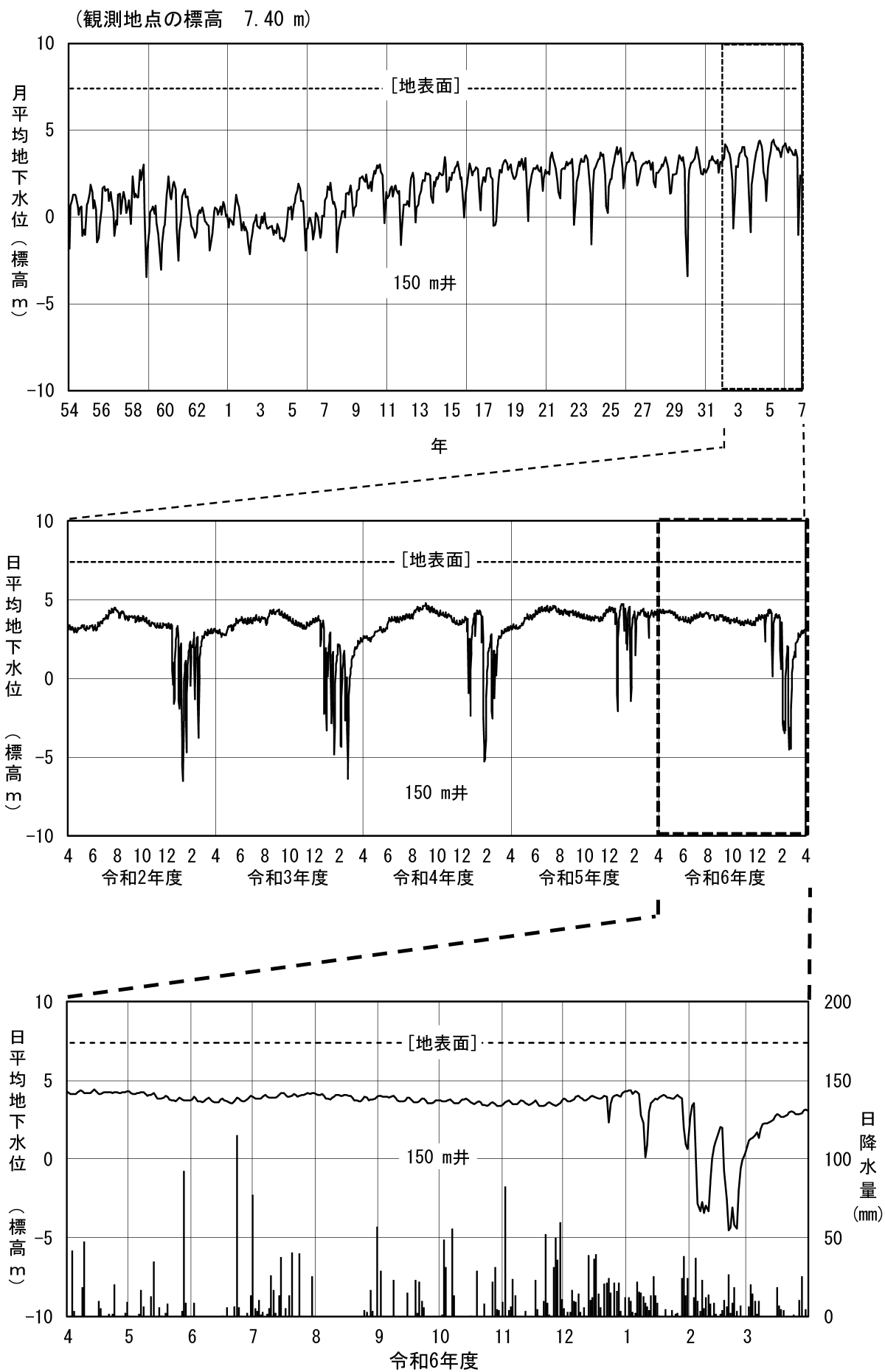
図 2-5 (7) 地下水位変動図 (④金沢市東力町)
