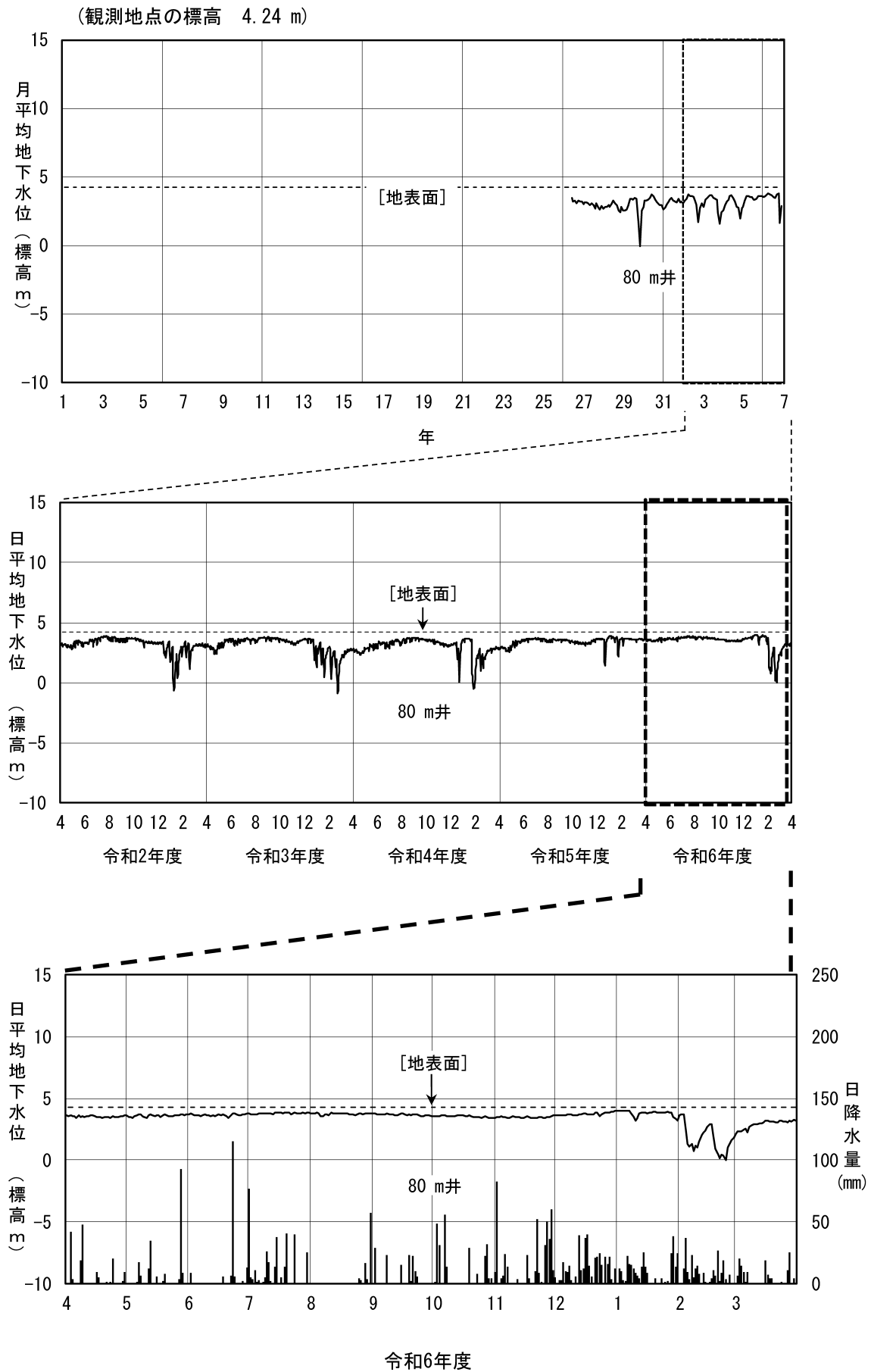
図 2-6 (7) 地下水位変動図 (⑫金沢市下安原町)
