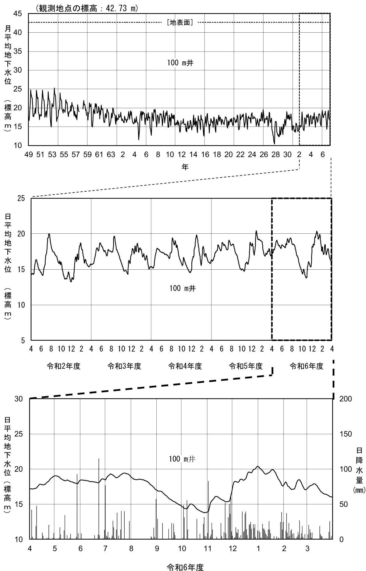
図 2-6(16) 地下水位変動図 (㊶白山市安吉町)
