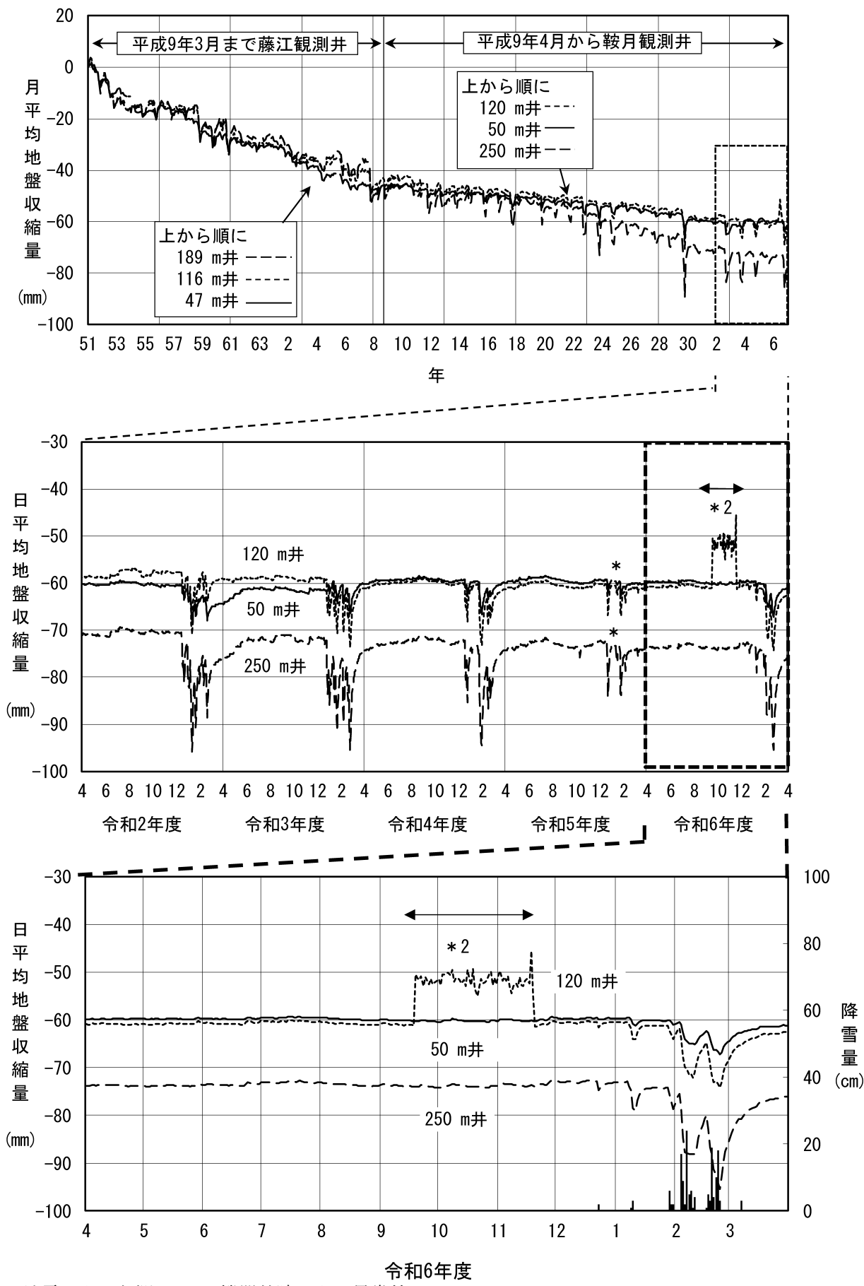
図 2-5 (2) 地盤収縮量変動図 (①金沢市鞍月)
