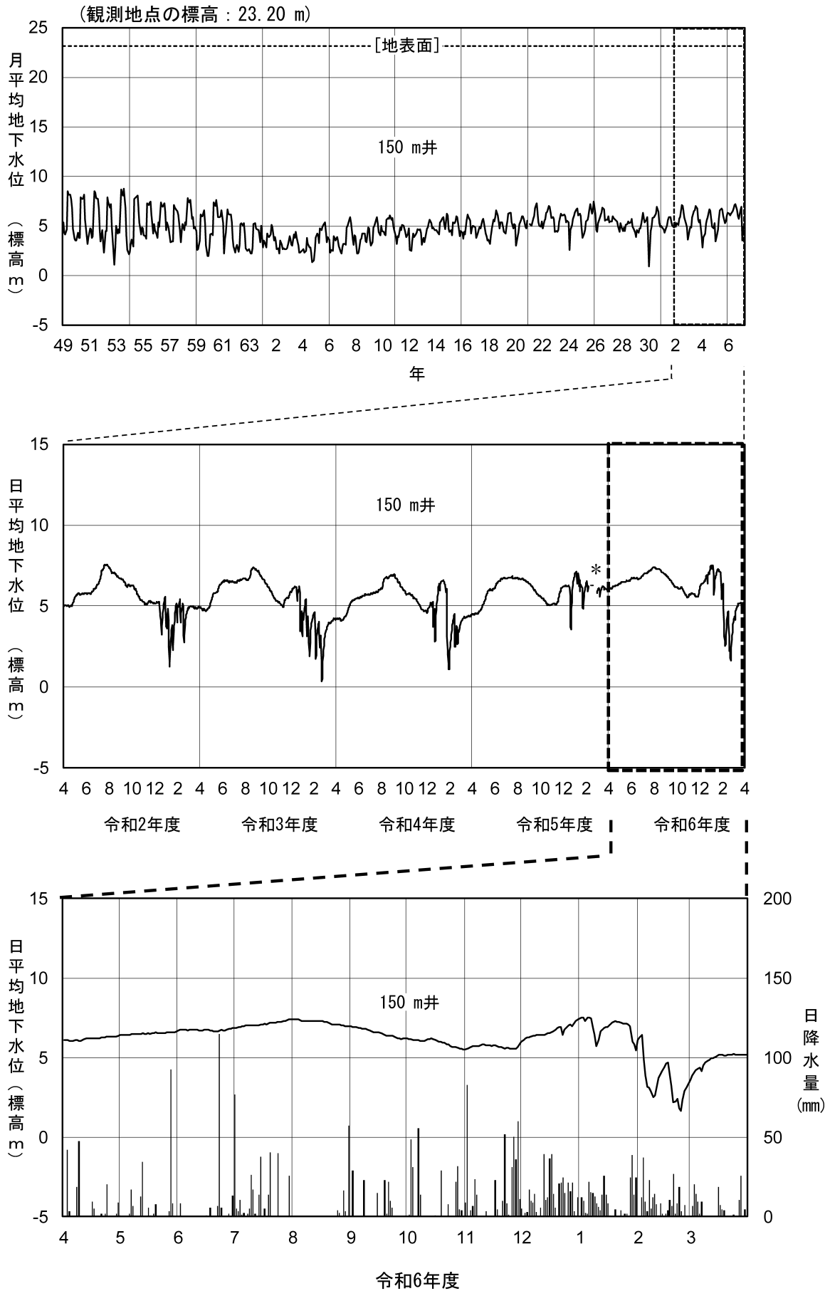
図 2-6(14) 地下水位変動図 (⑱野々市市太平寺)
