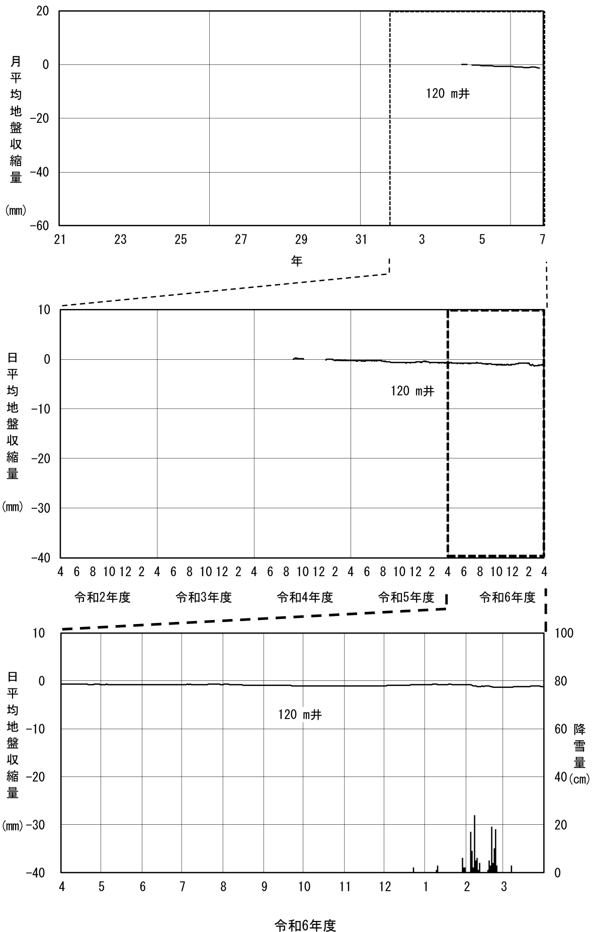
図 2-5(10) 地盤収縮量変動図 (⑤金沢市専光寺町(2))
