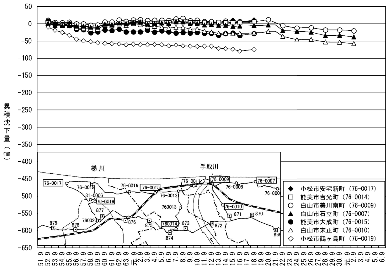
図 2-3(4) 主な水準点の累積地盤沈下量 (白山市～小松市)
