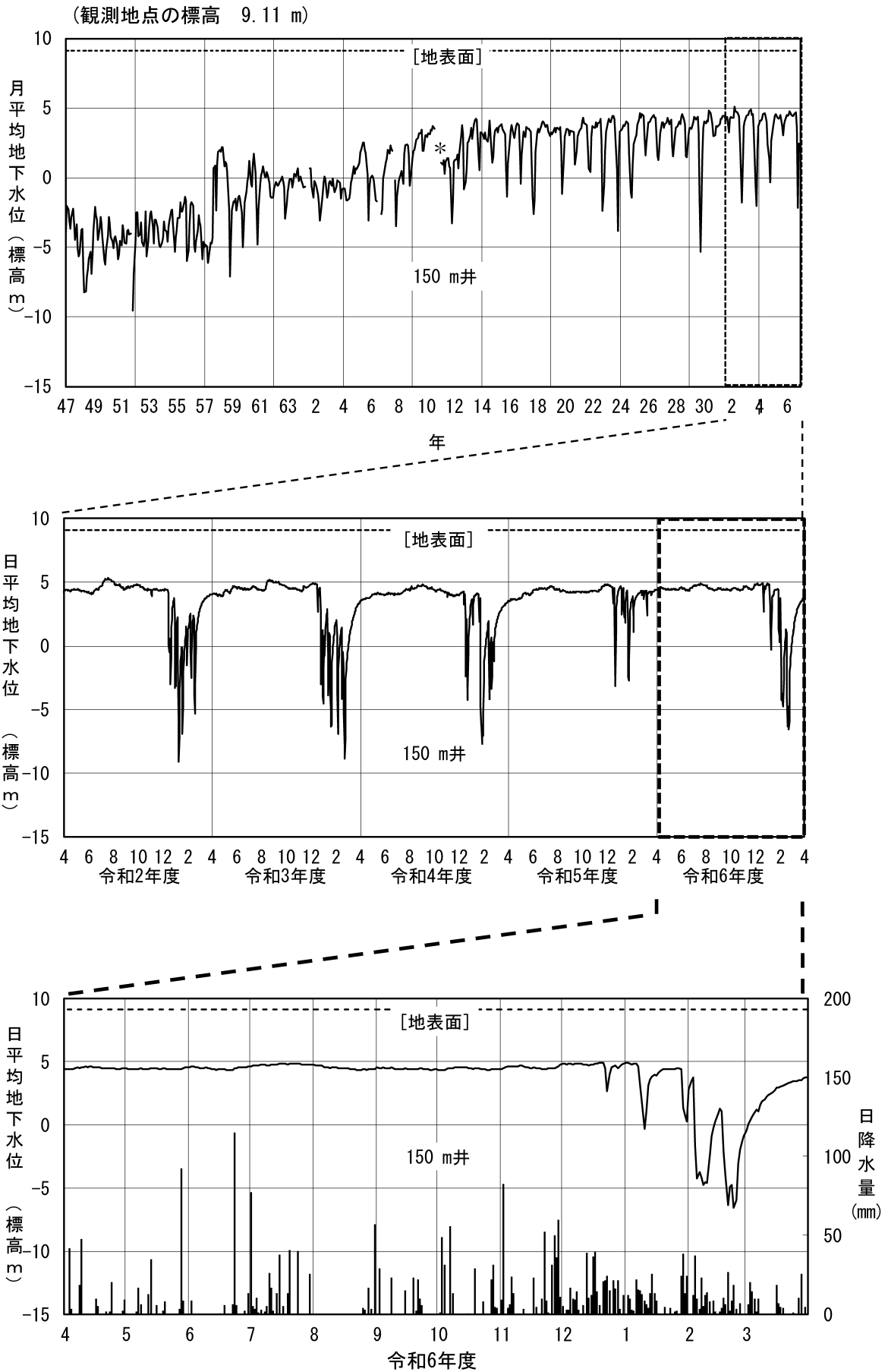
図 2-6(2) 地下水位変動図 (⑦金沢市昭和町)
