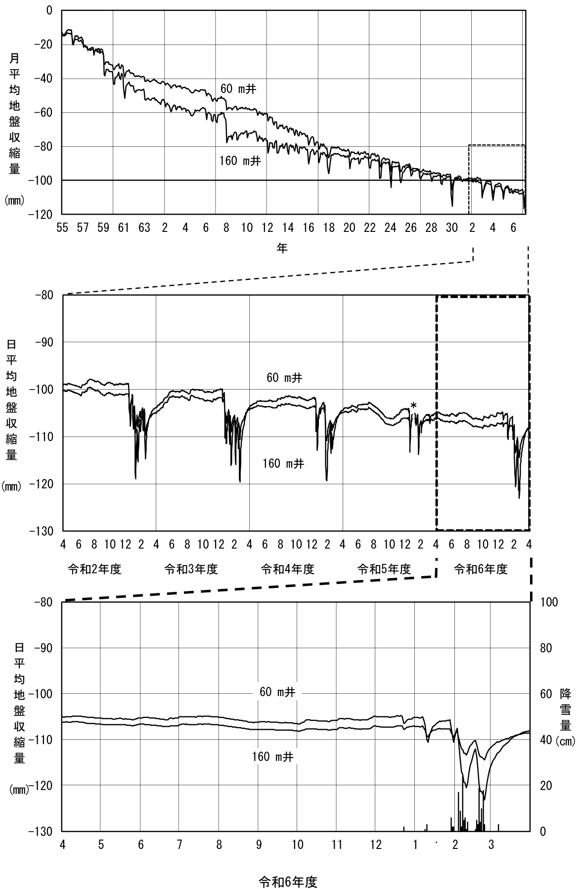
図 2-5 (6) 地盤収縮量変動図 (③金沢市浅野本町)
