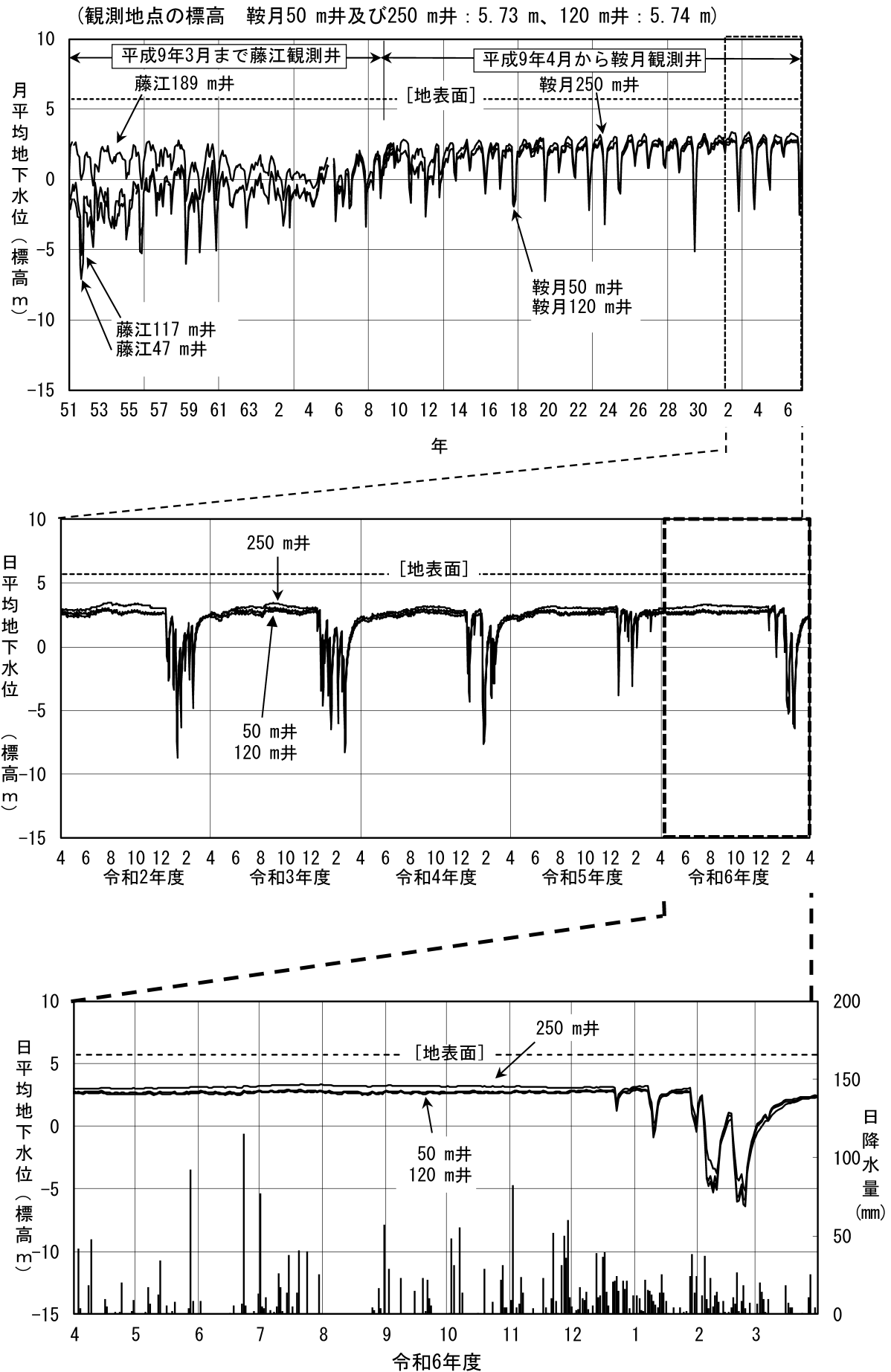
図 2-5 (1) 地下水位変動図 (①金沢市鞍月)
