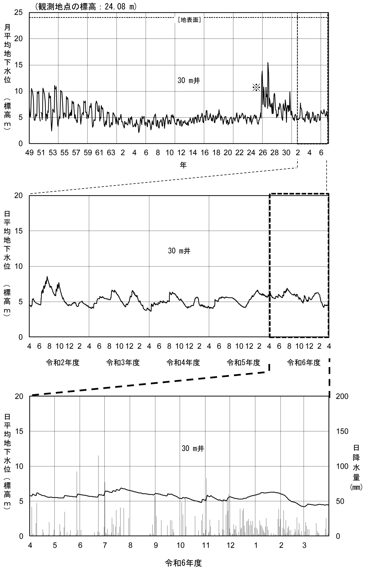
図 2-6(13) 地下水位変動図 (Ⓔ白山市末広)
