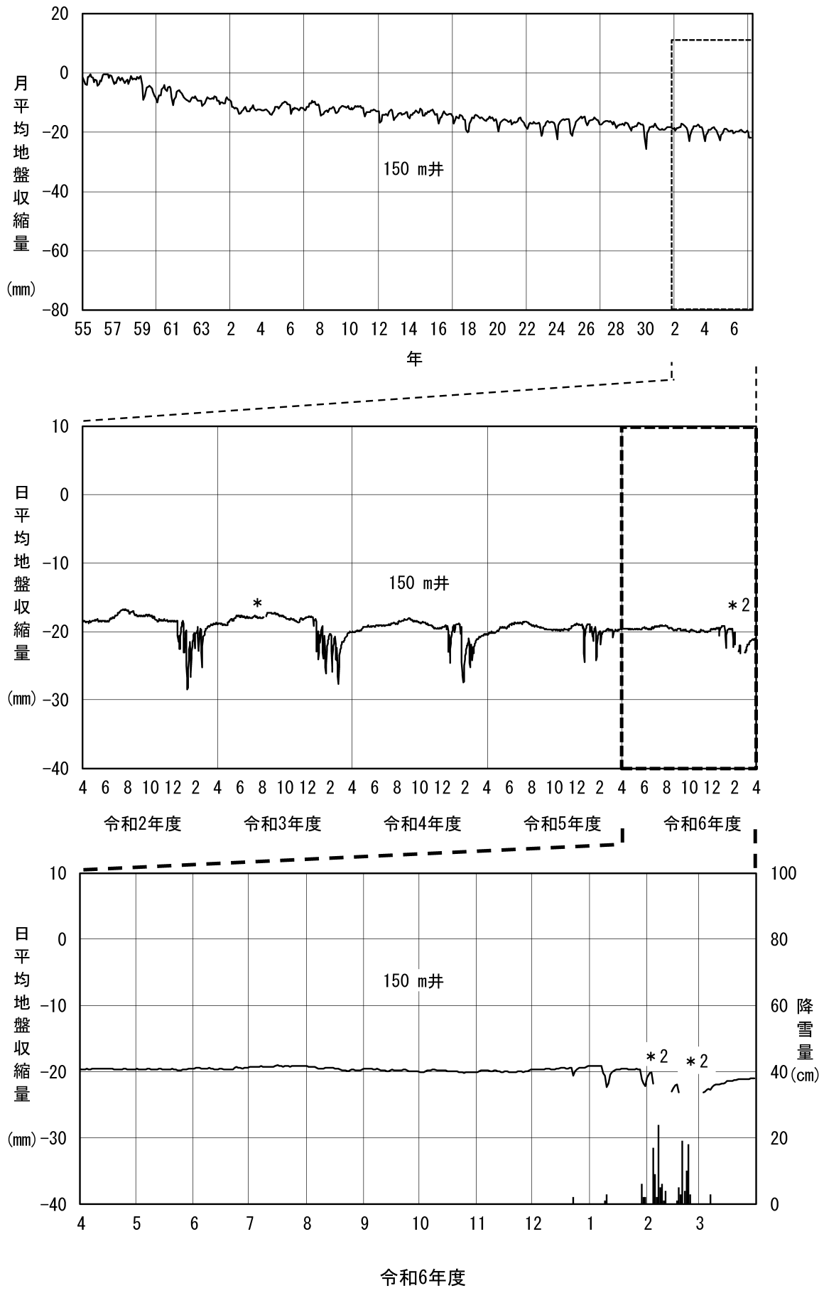
図 2-5 (8) 地盤収縮量変動図 (④金沢市東力町)
