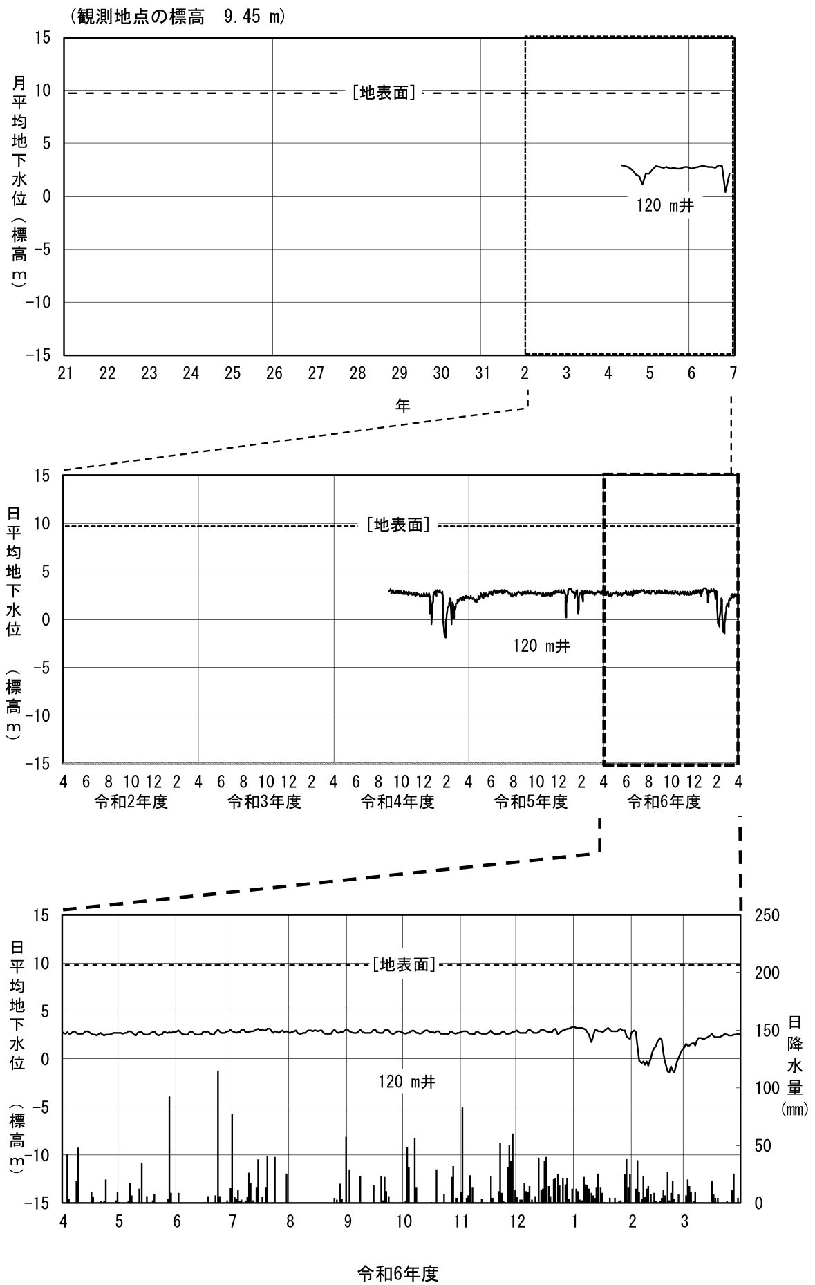
図 2-5 (9) 地下水位変動図 (⑤金沢市専光寺町(2))
