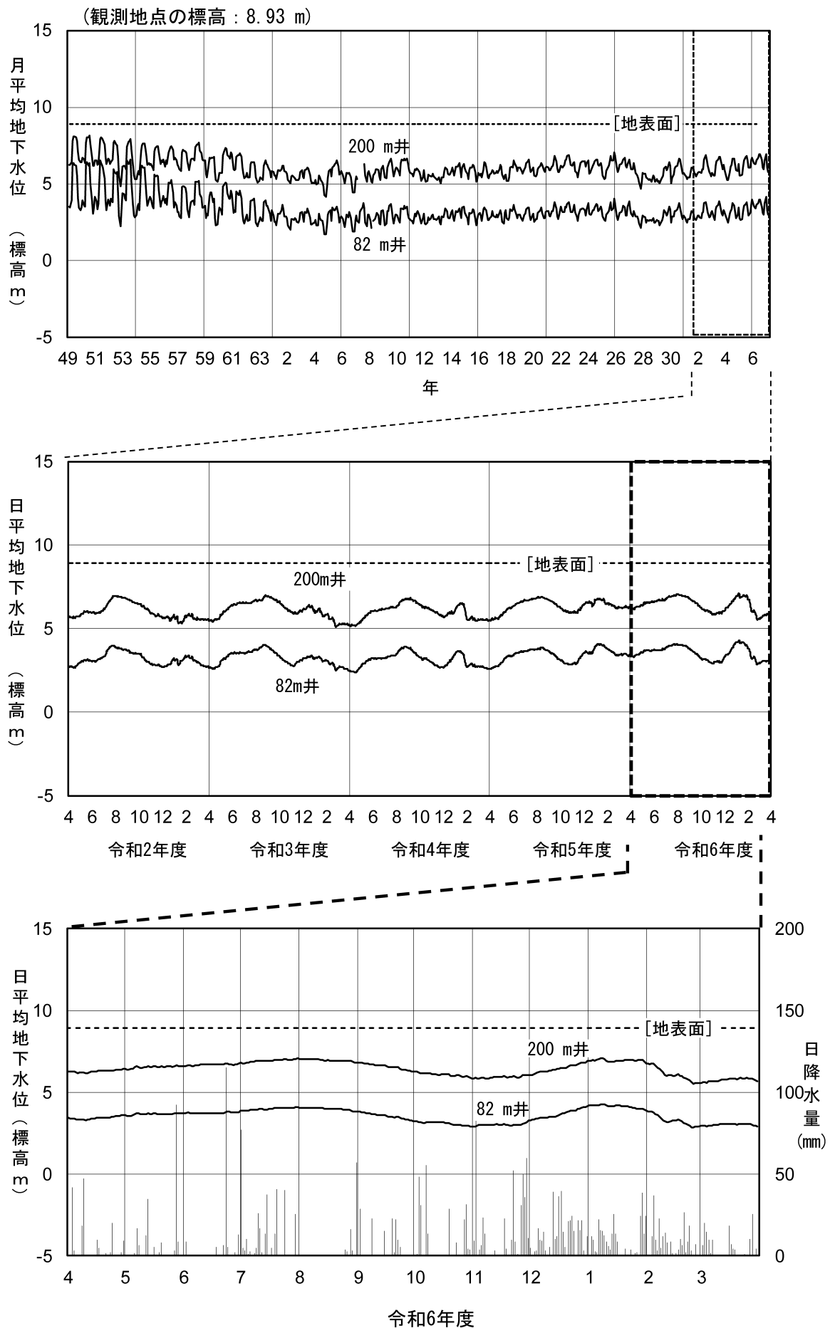
図 2-6(12) 地下水位変動図 (①白山市千代野西)
