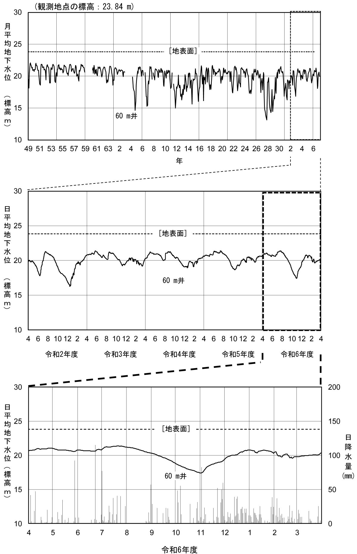
図 2-6(18) 地下水水位変動図 (㊸能美市北市)
