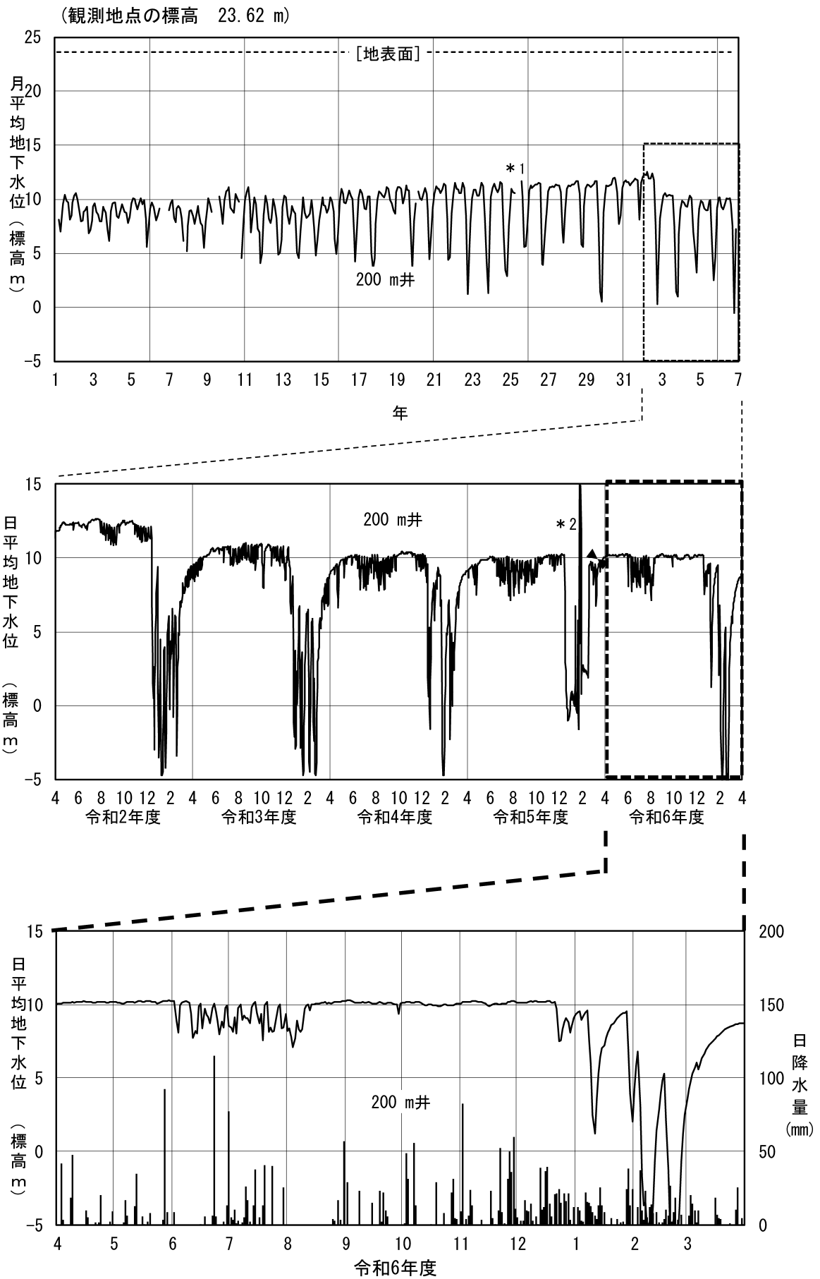
図 2-6 (3) 地下水位変動図 (⑧金沢市大手町)
