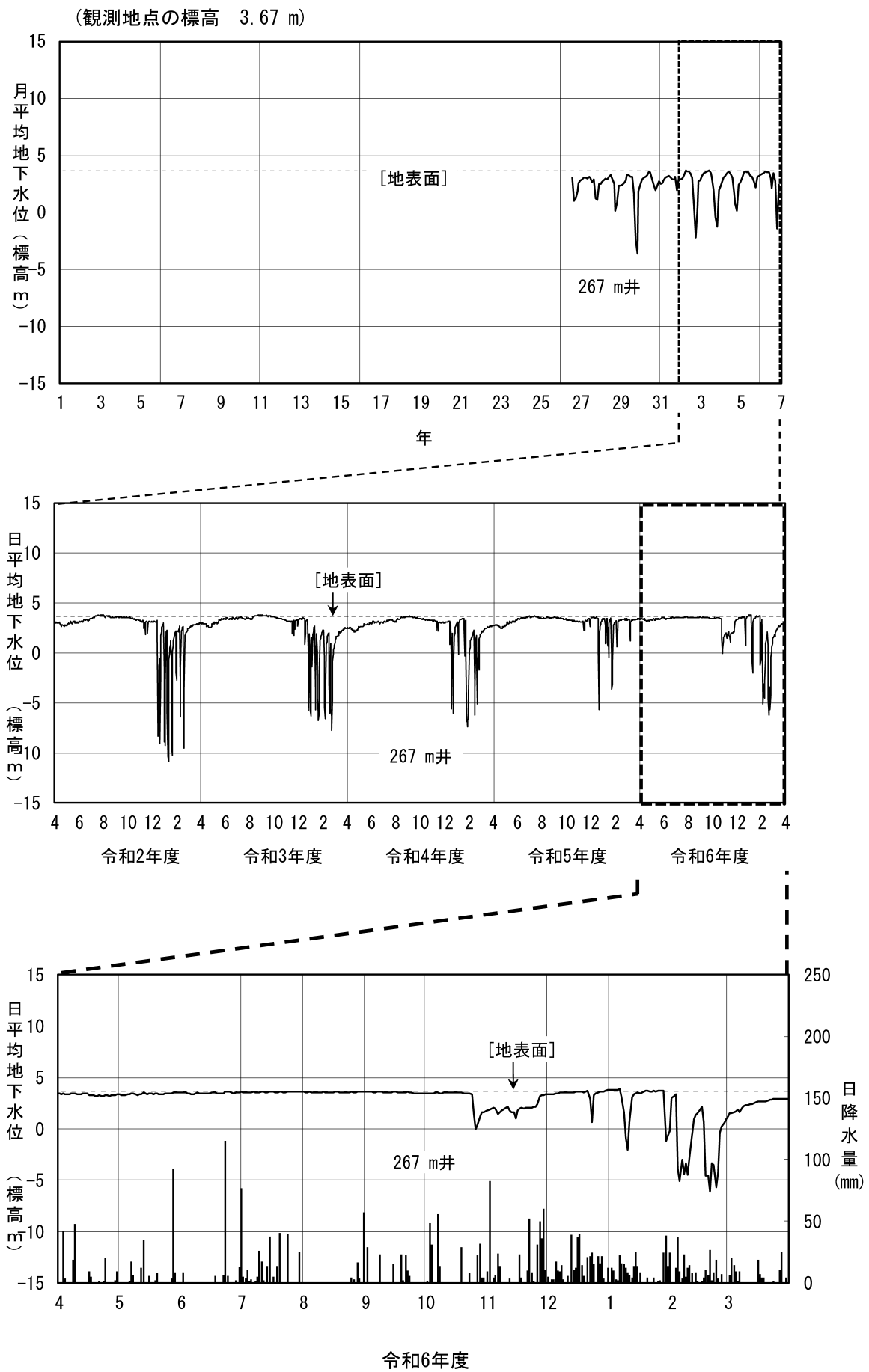
図 2-6(10) 地下水位変動図 (⑮金沢市専光寺町(1))
