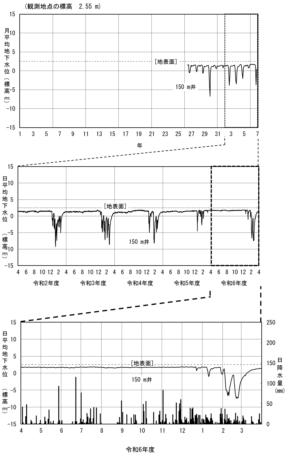
図 2-6(8) 地下水水位変動図 (⑬金沢市湊3丁目)
