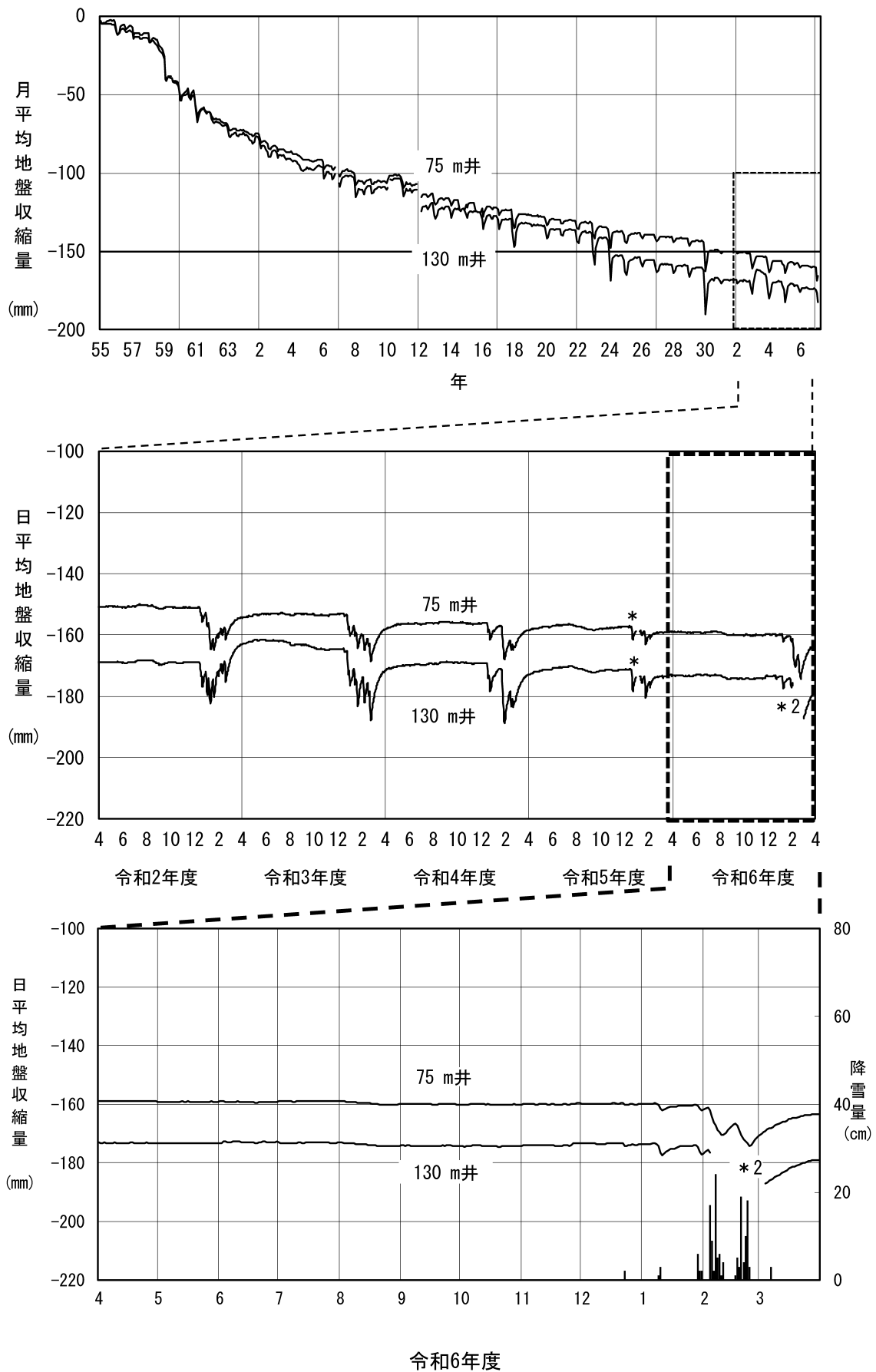
図 2-5 (4) 地盤収縮量変動図 (②金沢市須崎町)
