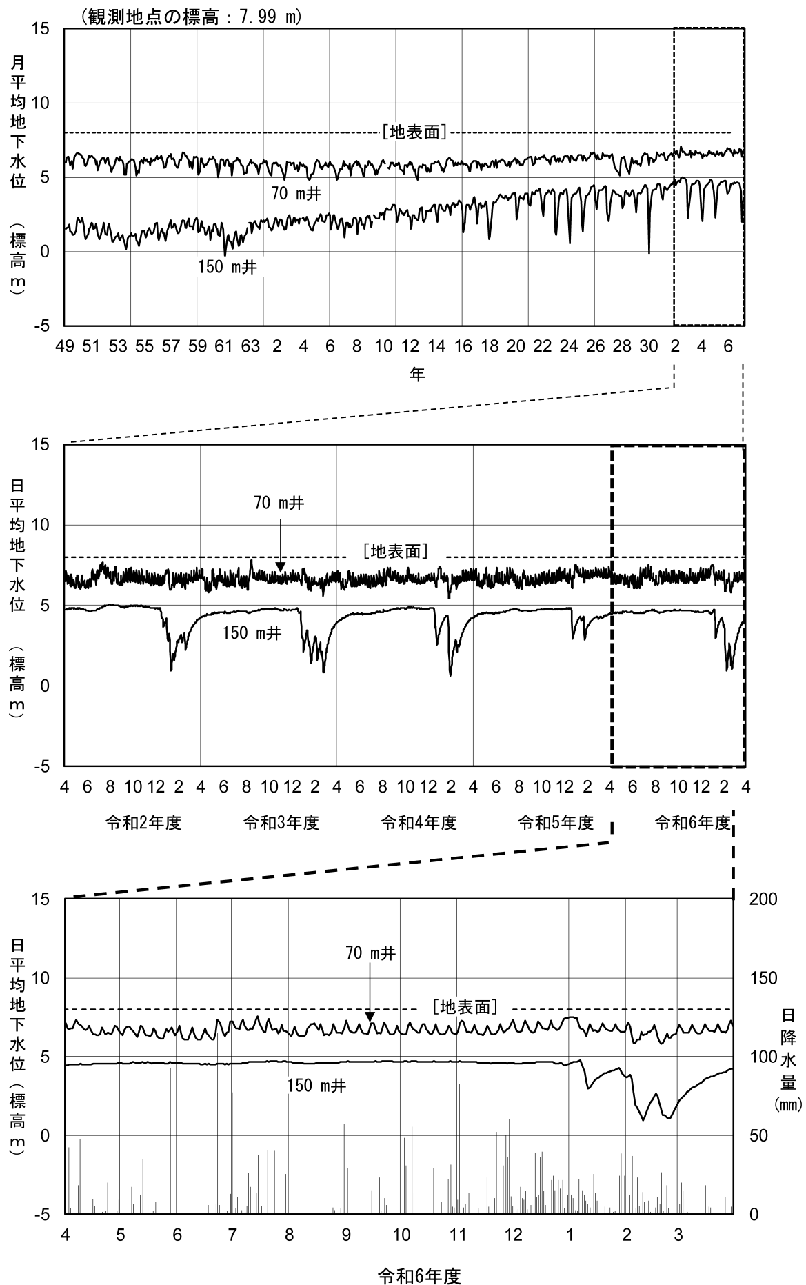
図 2-6(17) 地下水位変動図 (能美市赤井)
