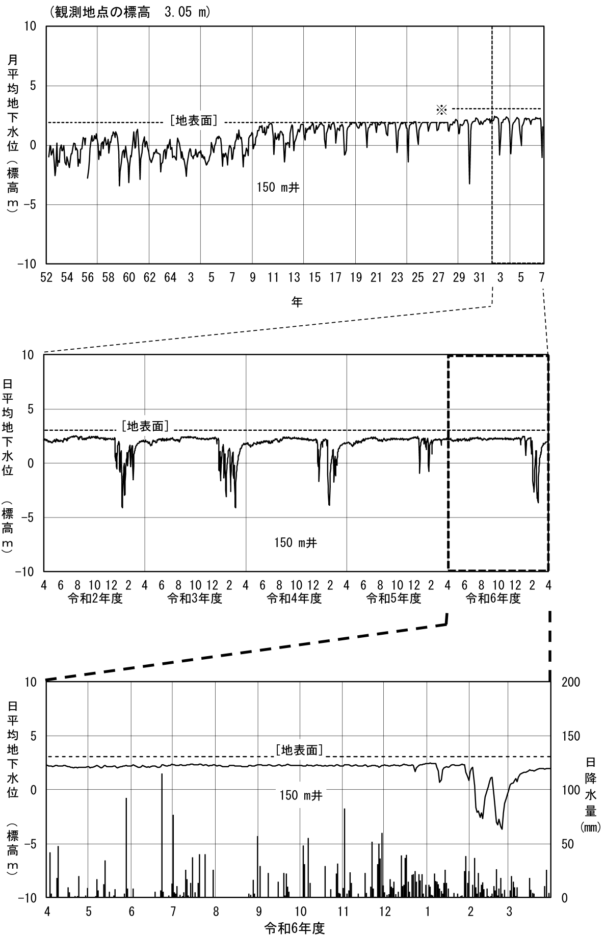
図 2-6(1) 地下水位変動図 (⑥金沢市金石東)
