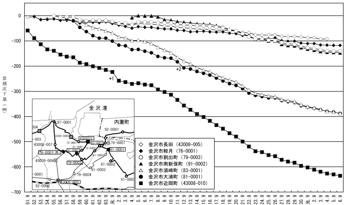
図 2-3(2) 主な水準点の累積地盤沈下量 (金沢市近郊)
