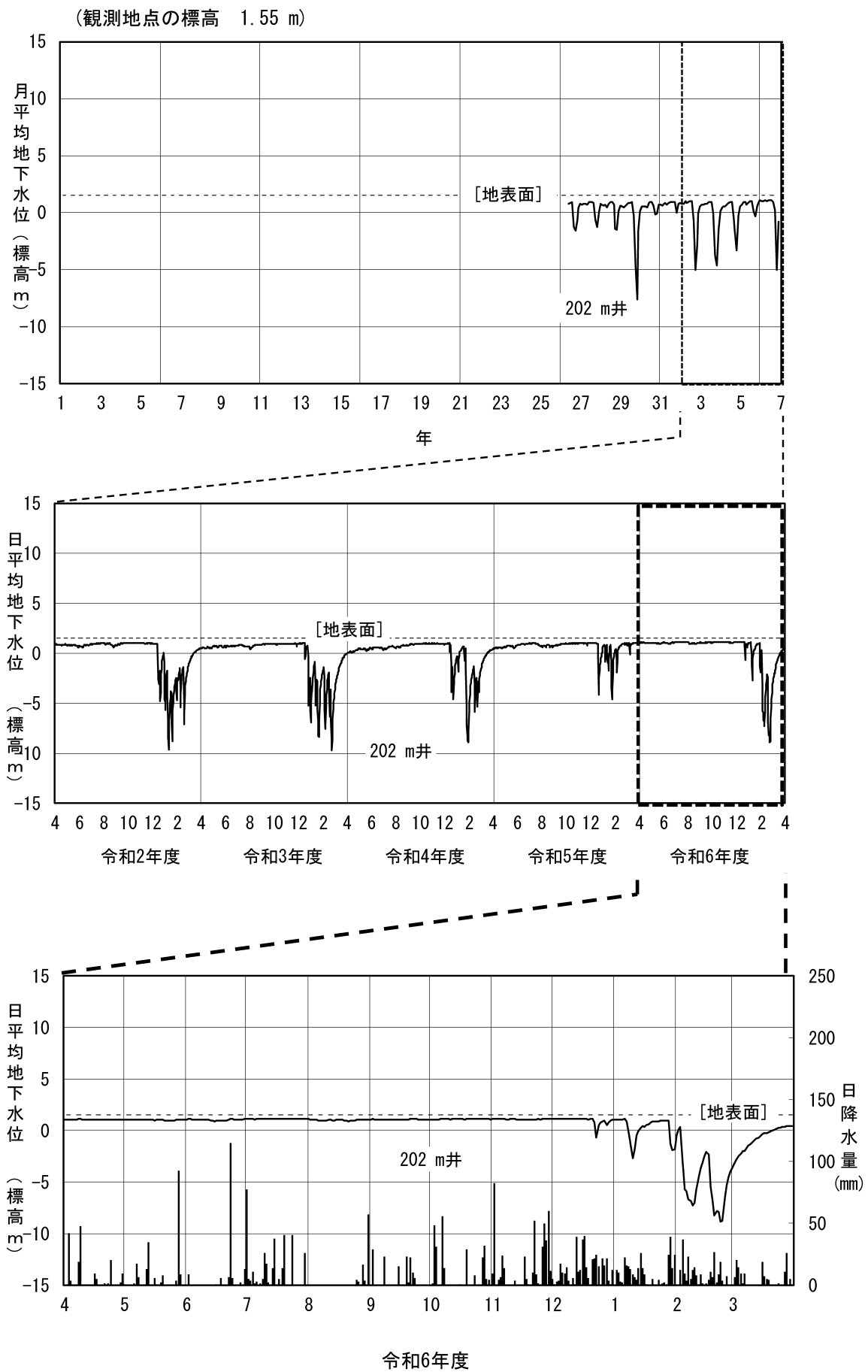
図 2-6(9) 地下水位変動図 (⑭金沢市東蚊爪町)
