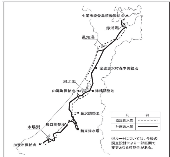
図11 県営水道の送水管耐震化事業
