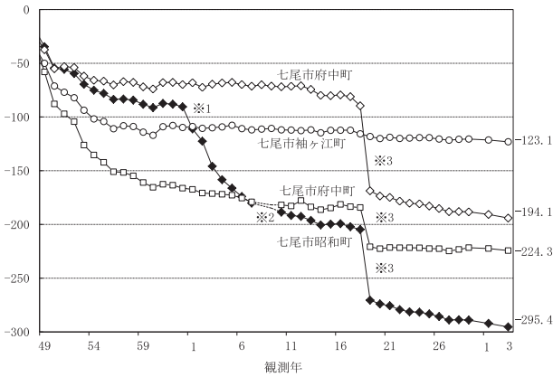
図2 七尾地域の主な地点の累計沈下量
