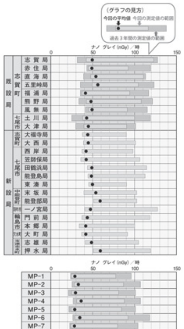
図39 線量率の測定結果（平成25年度分）
