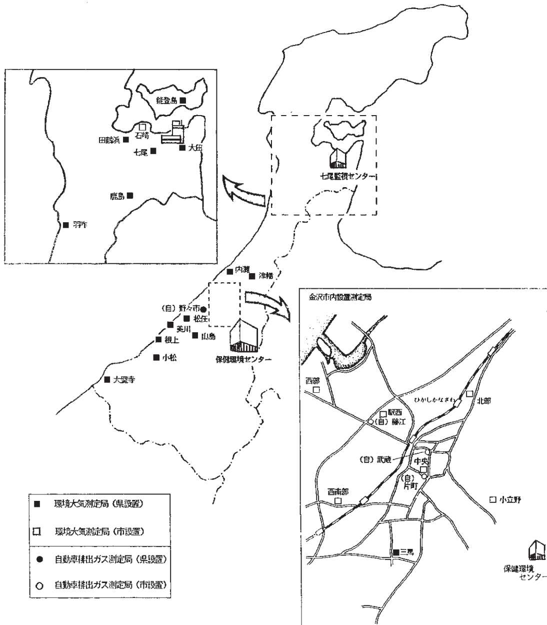
図18 県内における大気汚染常時監視網（平成25年3月現在）
