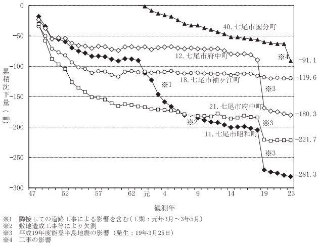
図2 七尾地域の主な地点の累計沈下量
