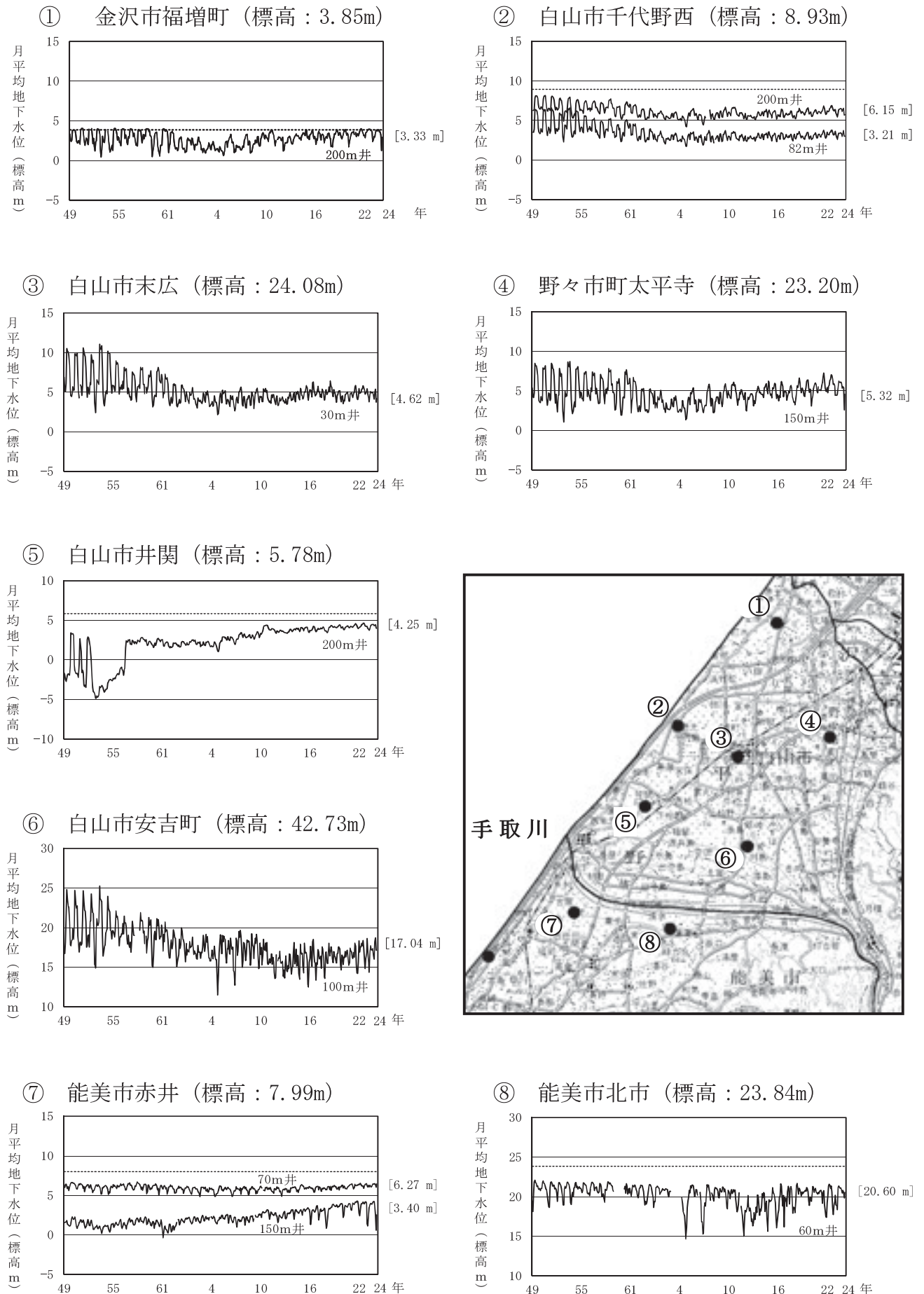
図4 手取川扇状地域における地下水位の変化
