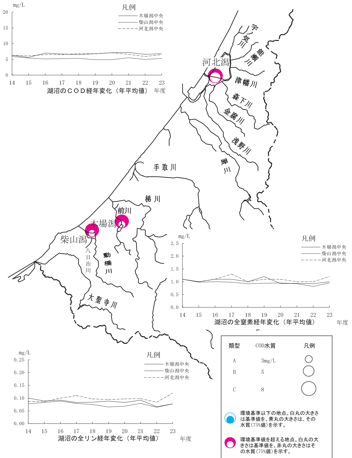
図15 生活環境の保全に関する環境基準達成状況と経年変化—湖沼— (CODの湖沼環境基準達成状況及びCOD、全窒素、全リン年平均値の経年変化)
