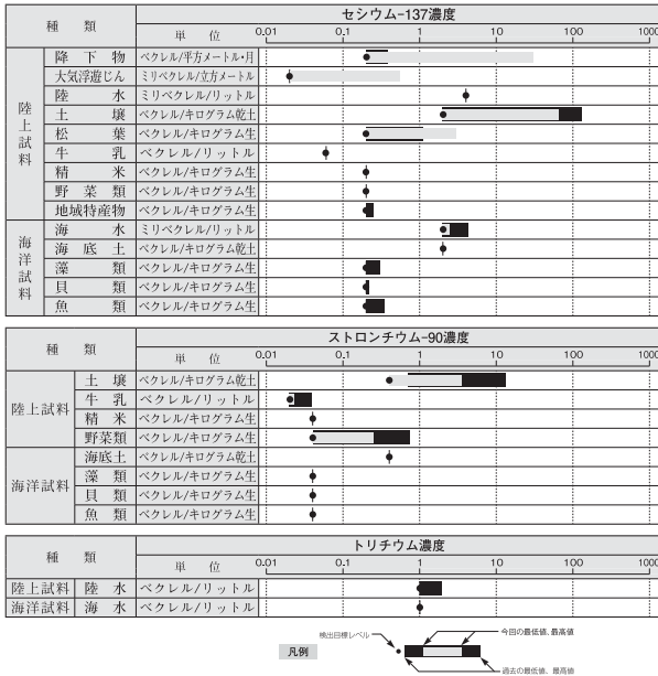
図38 環境試料中のセシウム-137、ストロンチウム-90、トリチウムの測定結果（平成23年度分）
