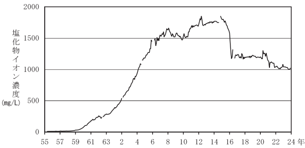
図5 能美市道林観測井の塩化物イオン濃度の経年変化(昭和56年～平成23年度)
