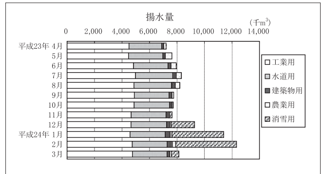
図8 月別の地下水揚水量(平成23年度)
