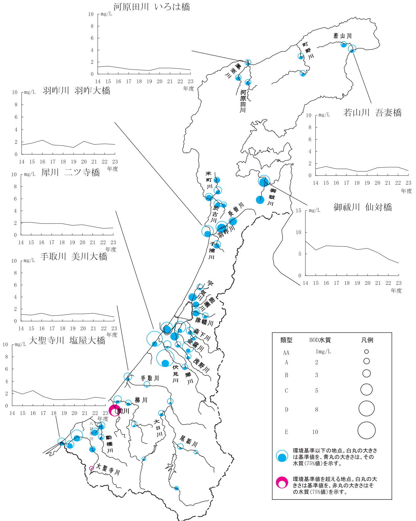
図14 生活環境の保全に関する環境基準達成状況と経年変化—河川— (BODの河川環境基準達成状況及び主要河川のBOD年平均値の経年変化)
