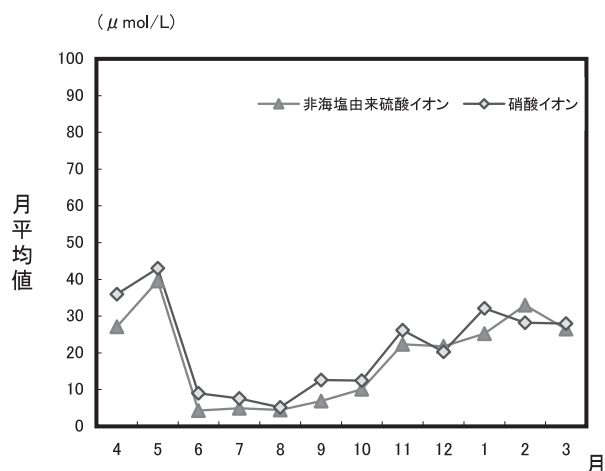
図27 平成24年度非海塩由来硫酸イオン及び硝酸イオンの経月変化 (月平均値)
