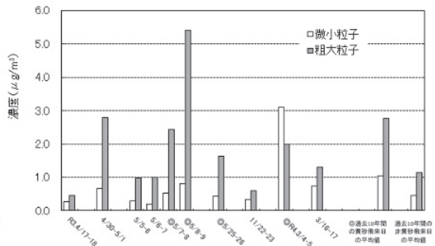
硝酸イオン
