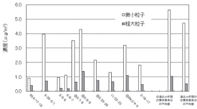
硫酸イオン
