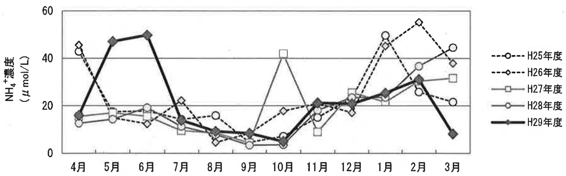
図6-4 月別 NH 4 + 濃度
