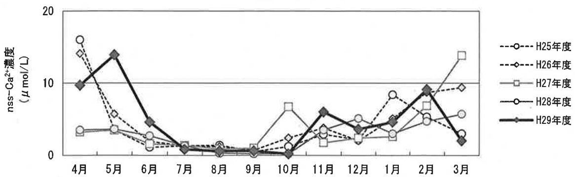
図6-5 月別 nss-Ca 2+ 濃度
