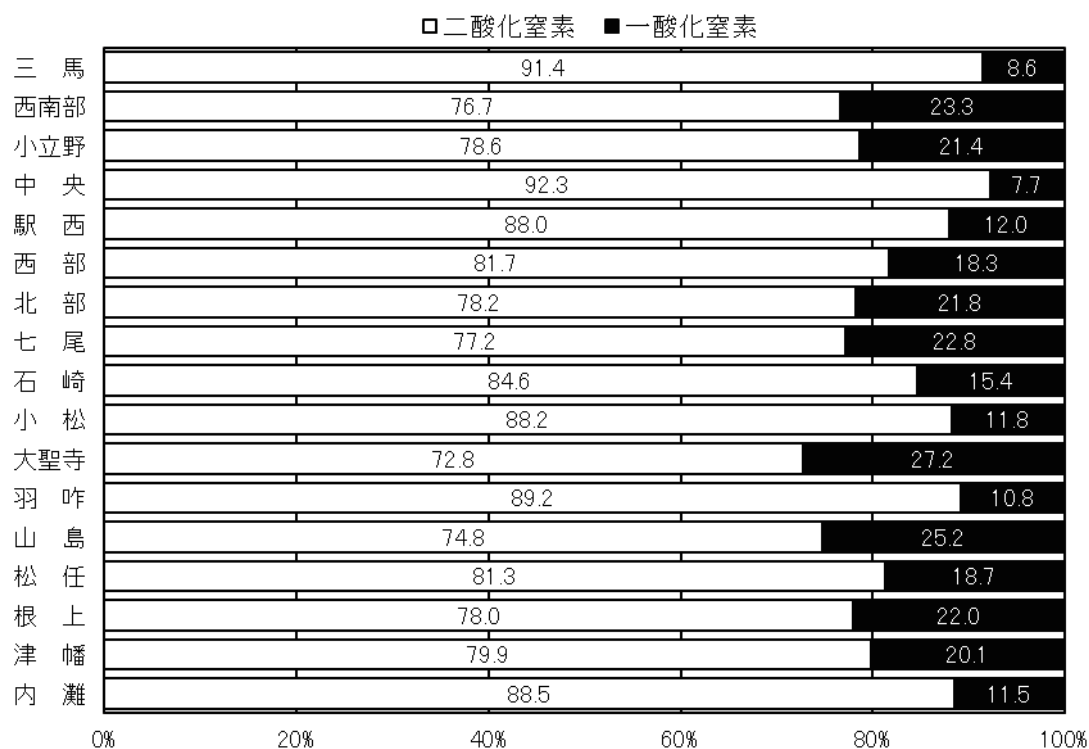
図 1-5 一般環境大気測定局における二酸化窒素と一酸化窒素の比率(平成 25 年度)
