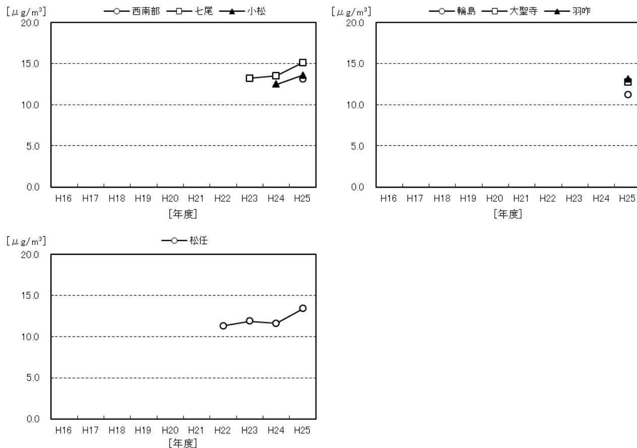
図 1-9 微小粒子状物質年平均値の経年変化
