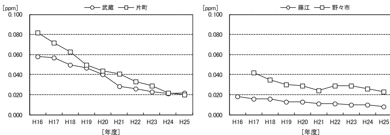
図 1-13 一酸化窒素年平均値の経年変化
