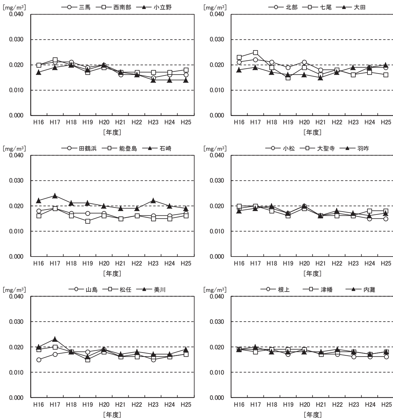
図1-8 10年間継続測定局における浮遊粒子状物質年平均値の経年変化
