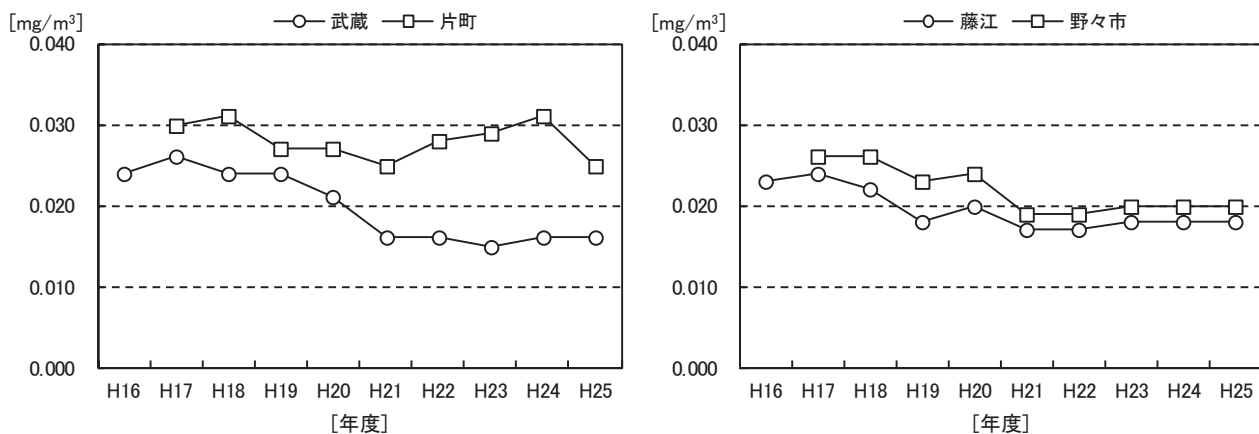
図1-15 浮遊粒子状物質年平均値の経年変化
