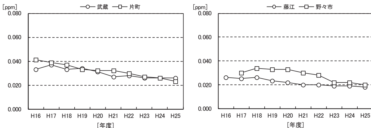
図1-12 二酸化窒素年平均値の経年変化
