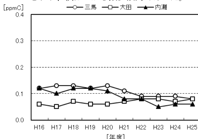
図 1-10 非メタン炭化水素の午前 6 時から 9 時における年平均値の経年変化
