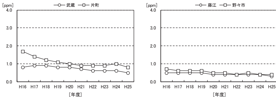
図 1-14 一酸化炭素年平均値の経年変化
