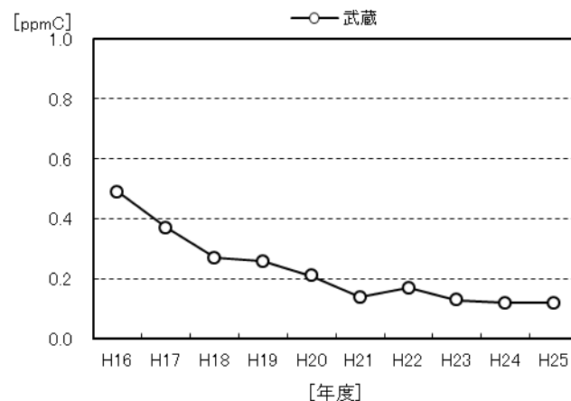
図 1-16 非メタン炭化水素の午前 6 時から 9 時における年平均値の経年変化
