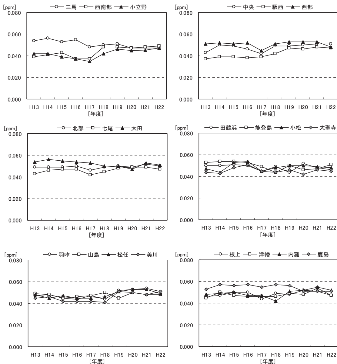
図 1-7 10 年間継続測定局における光化学オキシダント昼間の日最高 1 時間値年平均値の経年変化
