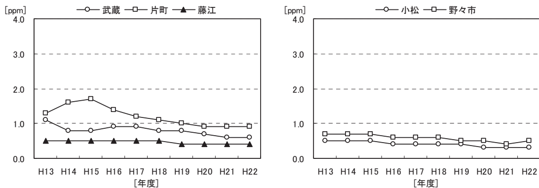
図 1-13 一酸化炭素年平均値の経年変化
