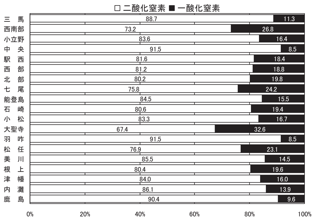
図 1-5 一般環境大気測定局における二酸化窒素と一酸化窒素の比率(平成 22 年度)
