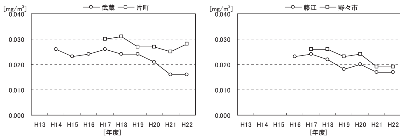
図1-14 浮遊粒子状物質年平均値の経年変化
