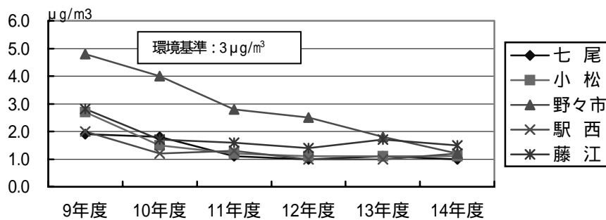
図4 - 4 ベンゼンの推移(年平均値)
