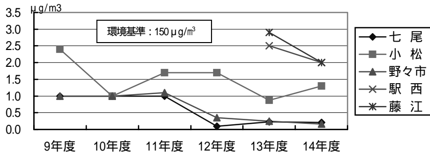
図4 - 1 ジクロロメタンの推移(年平均値)
