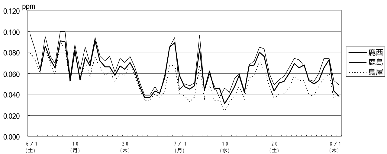
図 3 - 2 光化学オキシダント日最高値の推移
