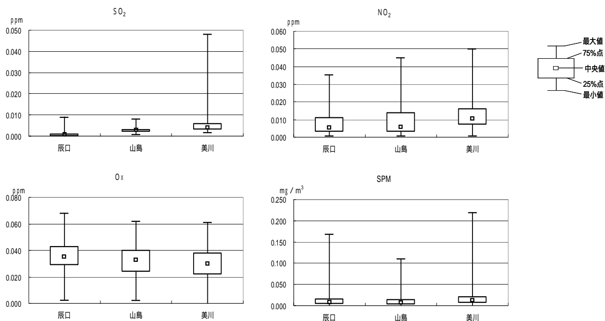
図3-4 近傍大気測定局の測定値との比較
