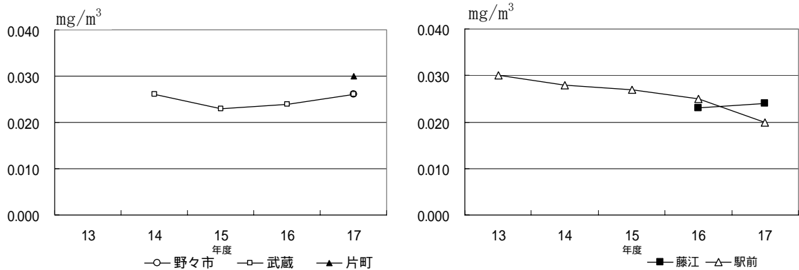
図2-21 浮遊粒子状物質濃度の経年変化
