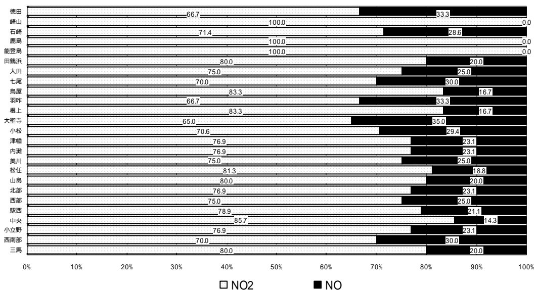
図2-6 一般環境大気測定局におけるNO 2 とNOの比率 (平成17年度)
