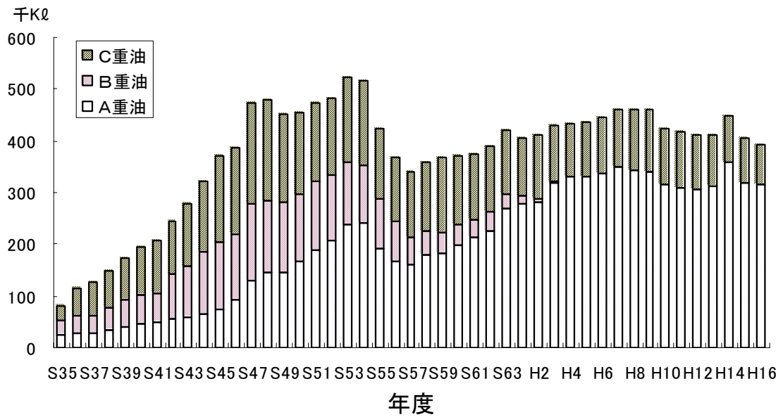
図 2 - 3 石川県における重油販売量の推移
