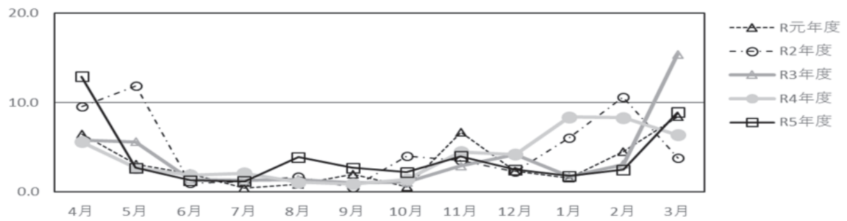
图 6-5 月别 nss- \text{Ca}^{2+} 浓度
