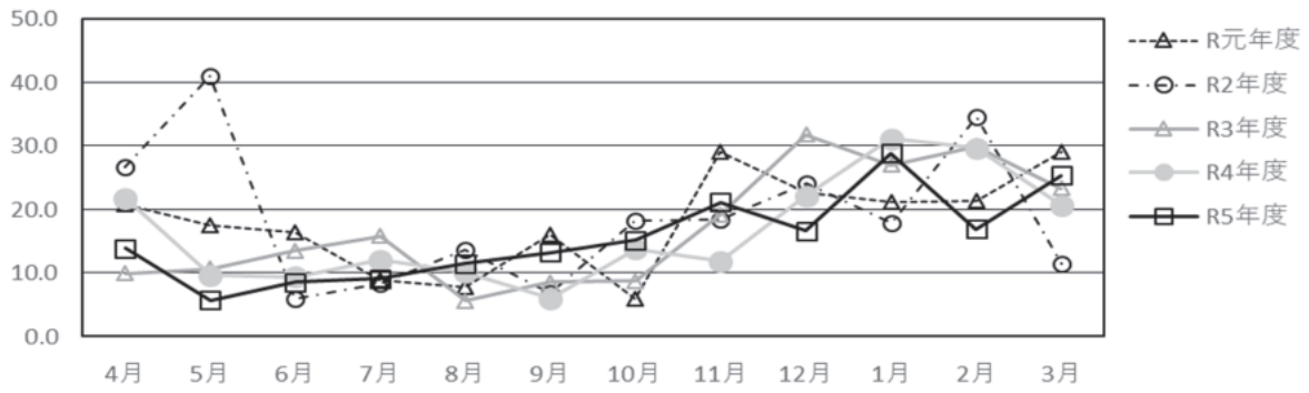
图 6-2 月别 \text{NO}_3^- 浓度
