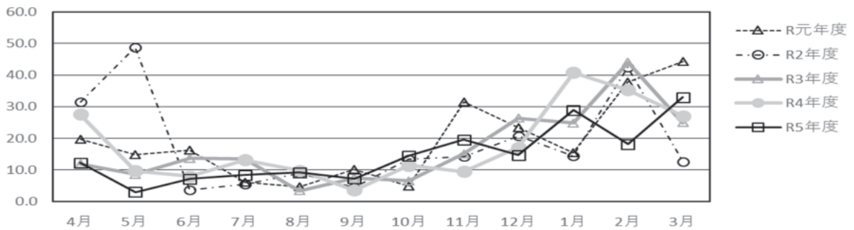
图 6-4 月别 \text{NH}_4^+ 浓度
