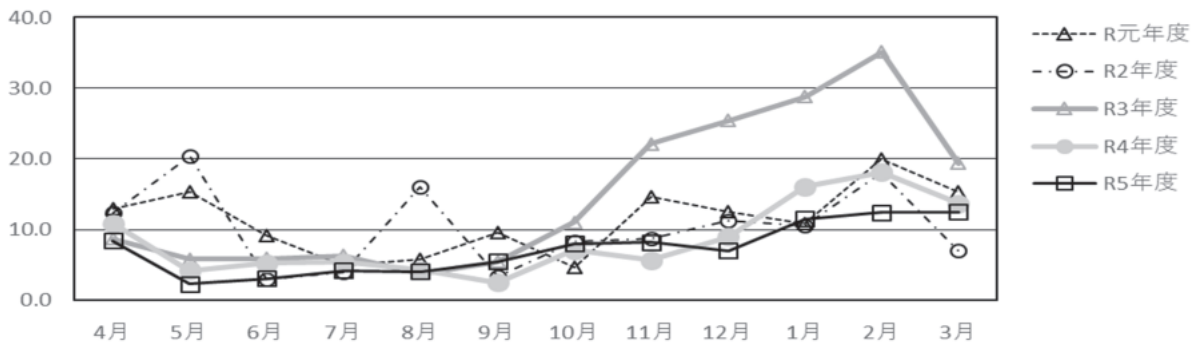
图 6-3 月别 nss- \text{SO}_4^{2-} 浓度
