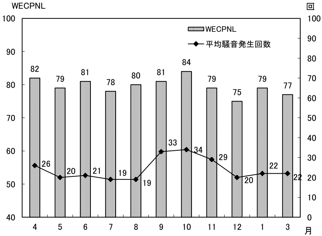
図-10 常時測定点における月別1日平均騒音発生回数とWECPNL (No. 1 小松市小島町)
