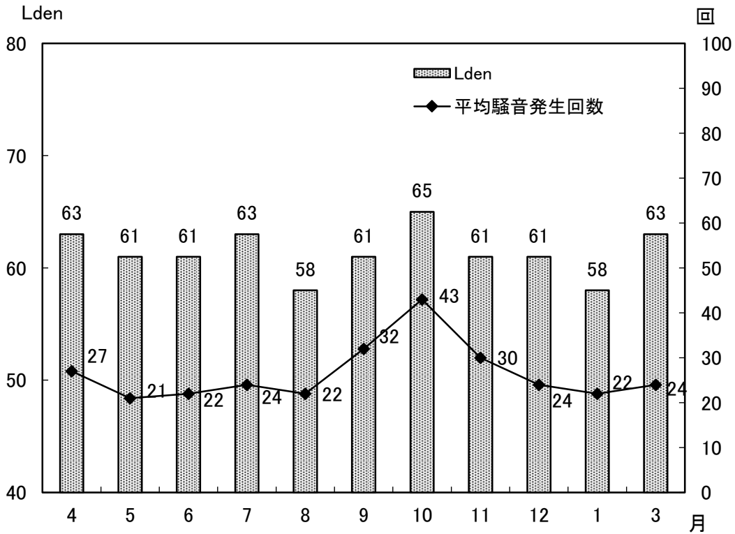
図-6 常時測定点における月別1日平均騒音発生回数とLden (No.2 加賀市伊切町)
