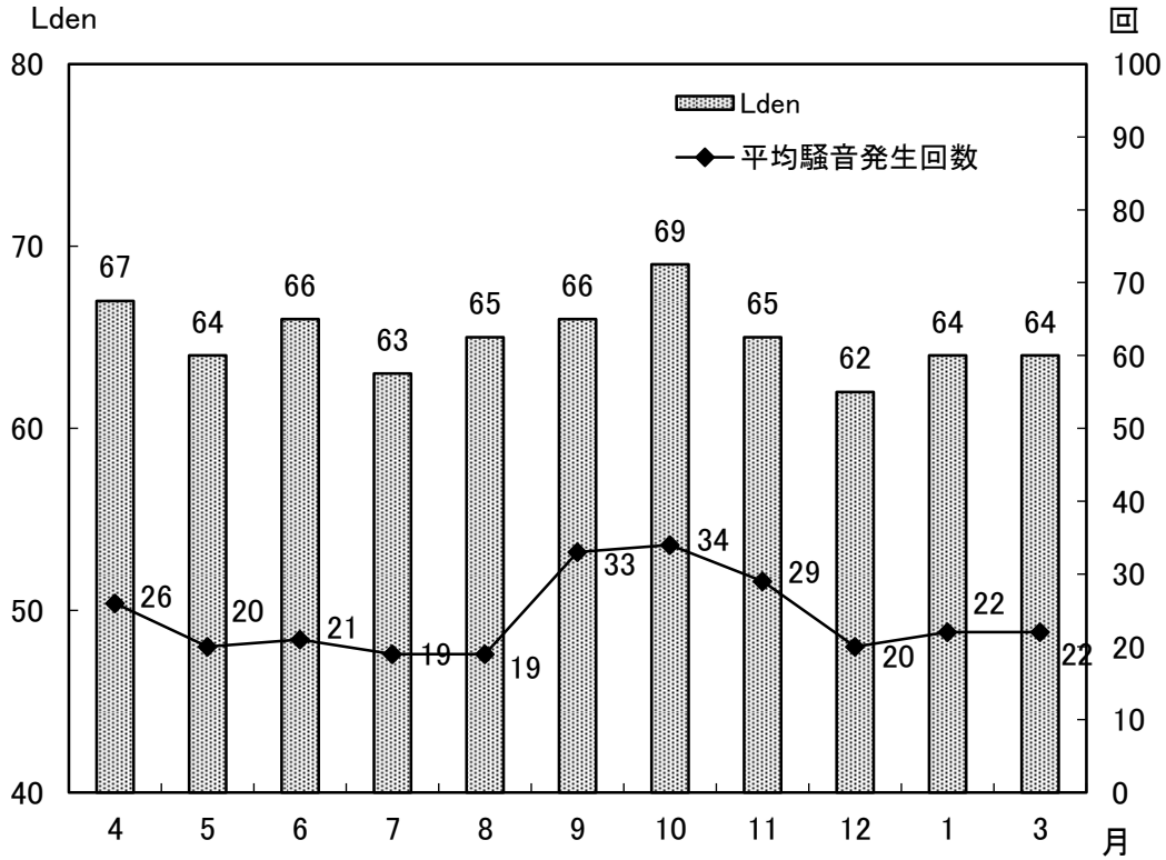
図-5 常時測定点における月別1日平均騒音発生回数とLden (No.1 小松市小島町)
