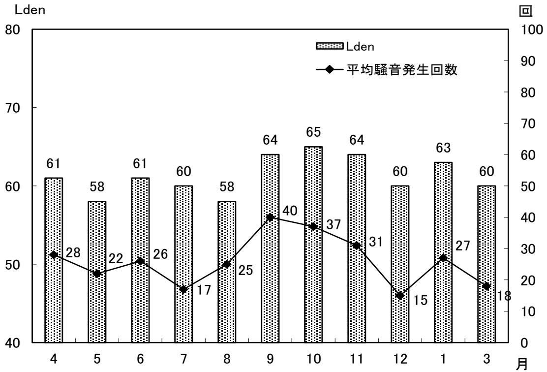
図-5 常時測定点における月別1日平均騒音発生回数とLden (No.1 小松市小島町)
