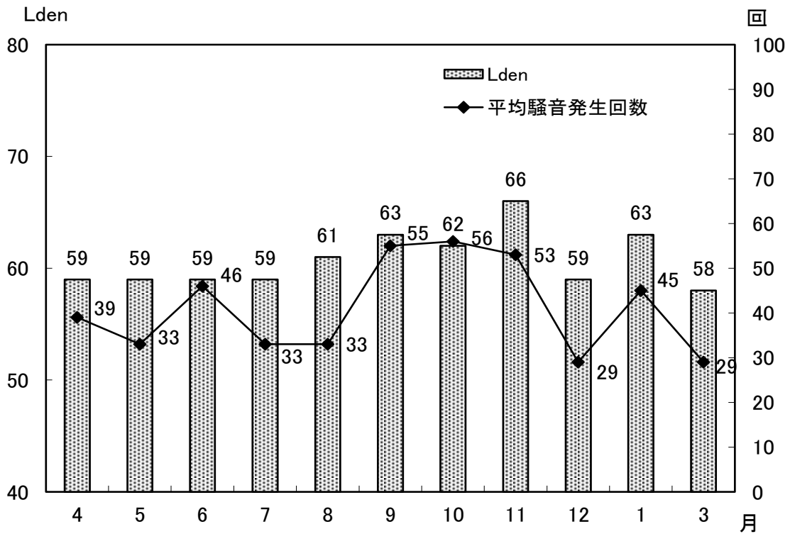
図-6 常時測定点における月別1日平均騒音発生回数とLden (No.2 加賀市伊切町)
