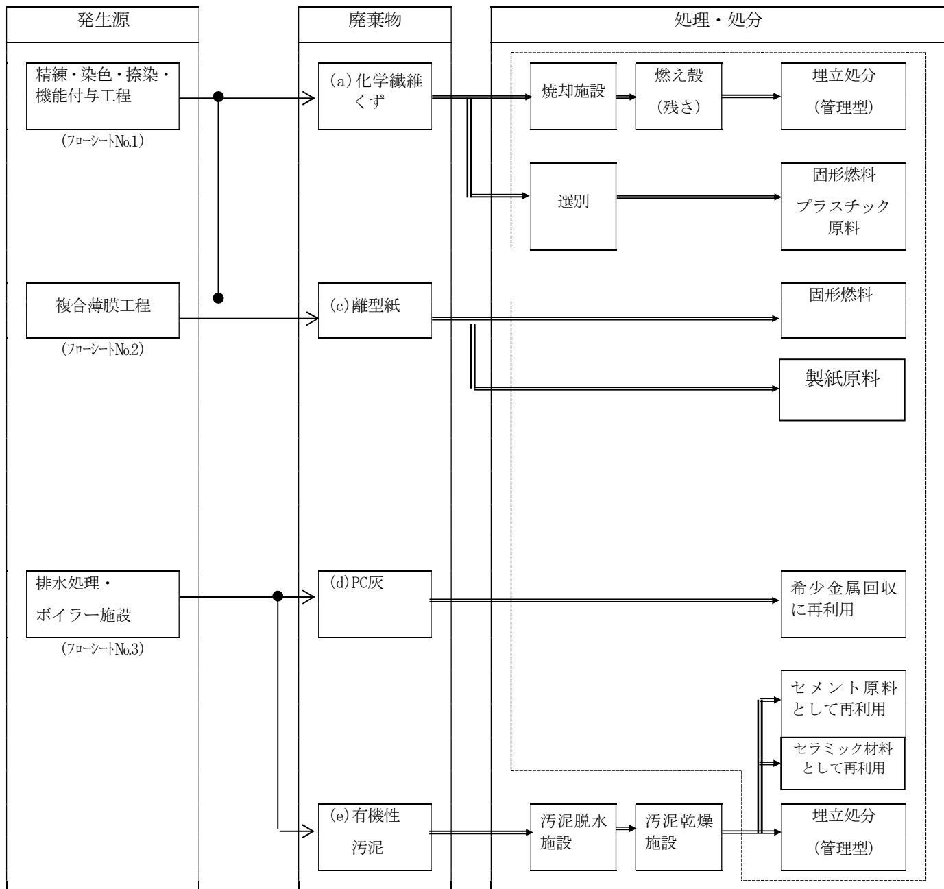
図 1. 廃棄物処理フローシート (現行)
