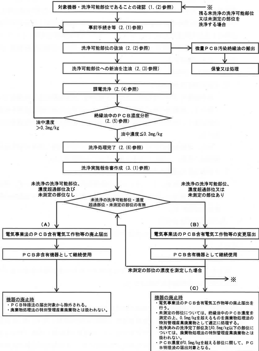
図 1-1 課電洗浄フロー図
