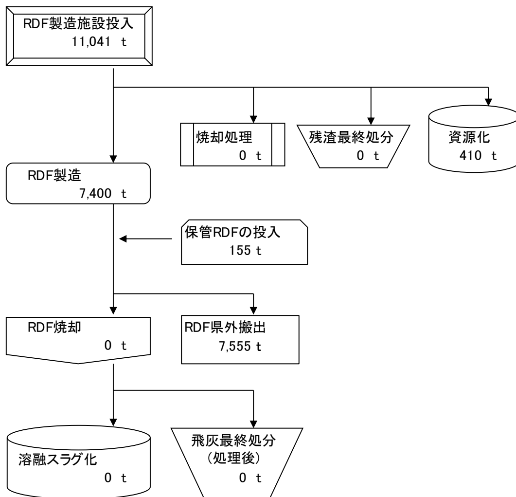
(参考) RDF 処理フロー (令和 6 年度実績)
