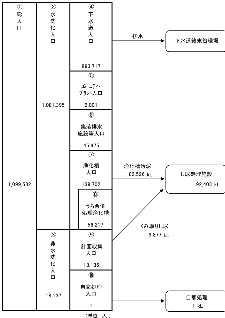
し尿処理フロー（令和 6 年度実績）
