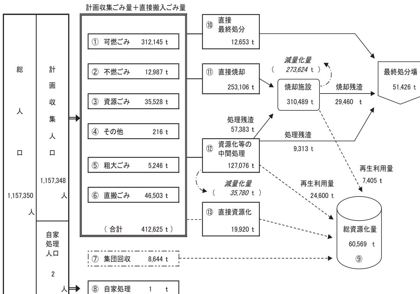
ごみ処理フロー（平成 27 年度実績）
