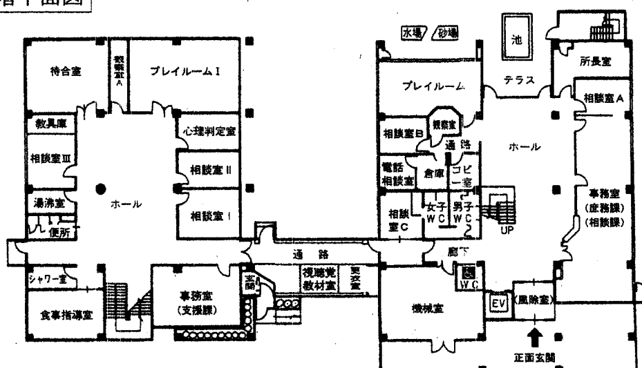
2 階平面図
