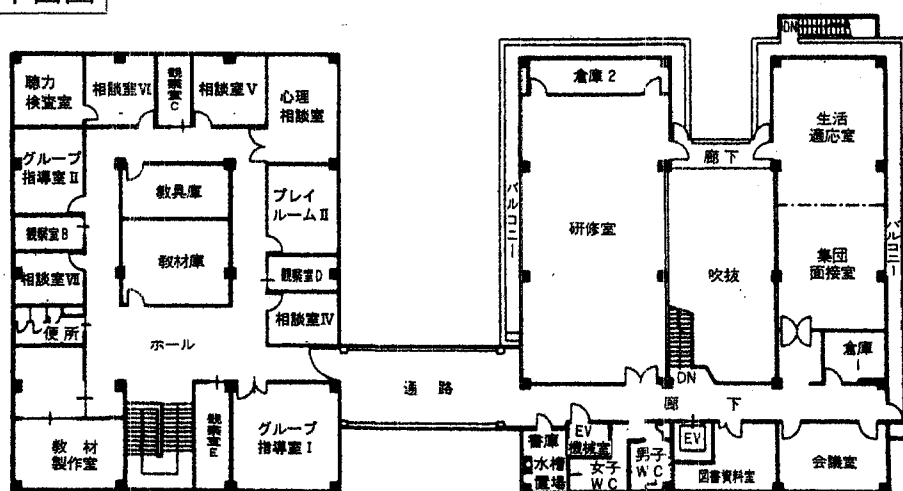
2 階平面図
