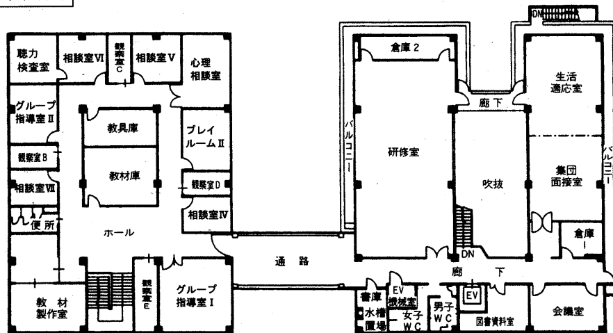
2階平面図
