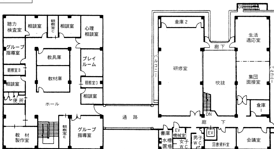
2階平面図
