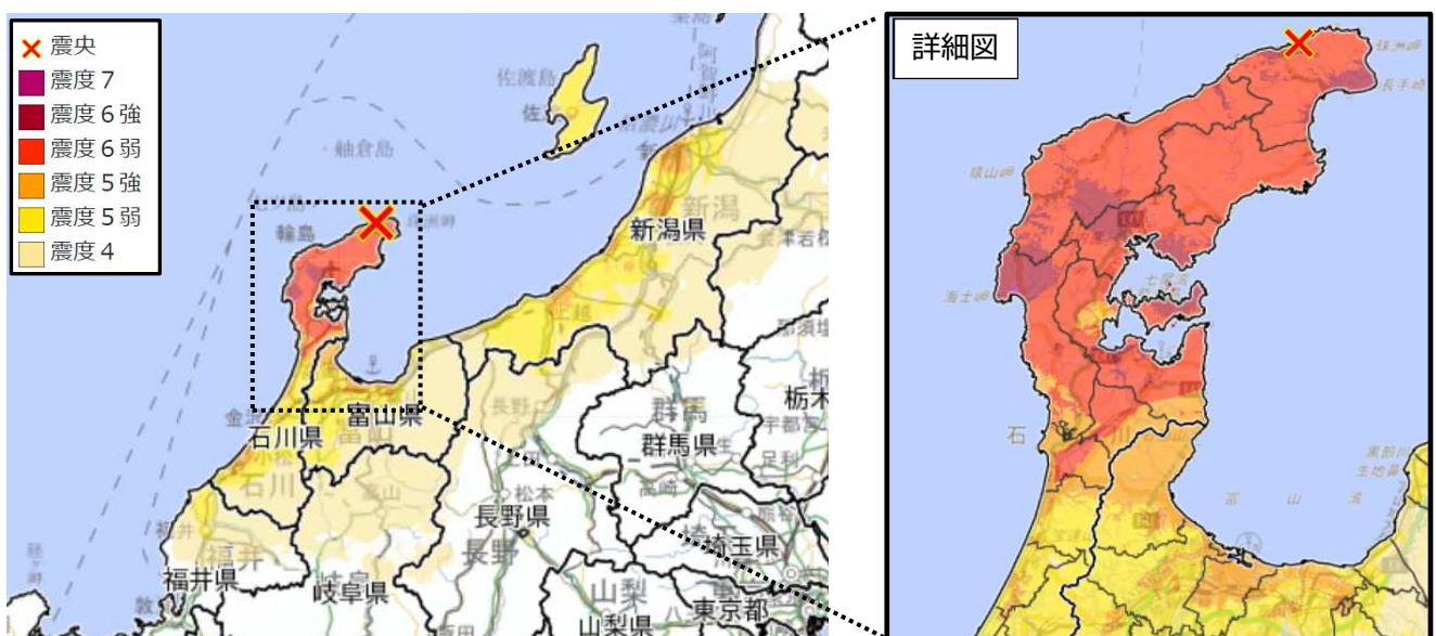
図1 震度分布図
