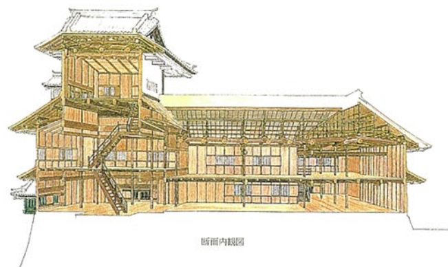
断面内観図
