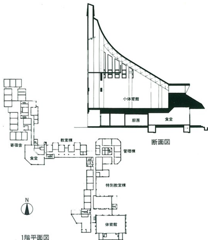
1階平面図
